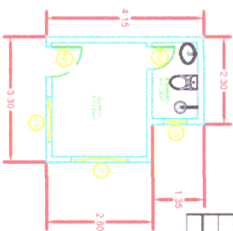
PLANTA BAIXA DA GUARITA
