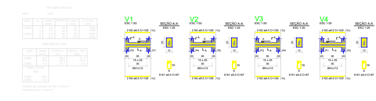
15 DETALHAMENTO DAS VIGAS BALDRAMES - ESTRUTURA DA CAIXA D'ÁGUA ESC.: INDICADA
