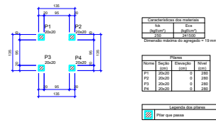
12 FORMA DOS PILARES - ESTRUTURA DA CAIXA D'ÁGUA ESC.: INDICADA
