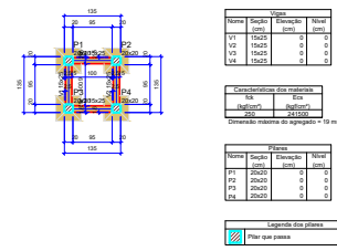
11 FORMA DA FUNDAÇÃO - ESTRUTURA DA CAIXA D'ÁGUA ESC.: INDICADA
