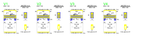
13 DETALHAMENTO DAS VIGAS DA LAJE - ESTRUTURA DA CAIXA D'ÁGUA ESC.: INDICADA
