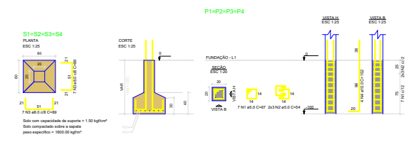
14 DETALHAMENTO DAS FUNDAÇÕES - ESTRUTURA DA CAIXA D'ÁGUA ESC.: INDICADA
