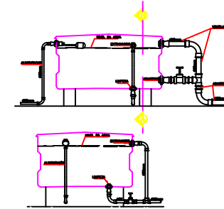
CORTE - A B
