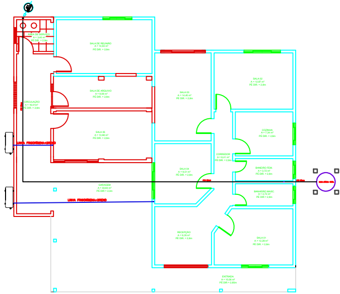
1 PLANTA HIDRÁULICA ESC. INDICADA
