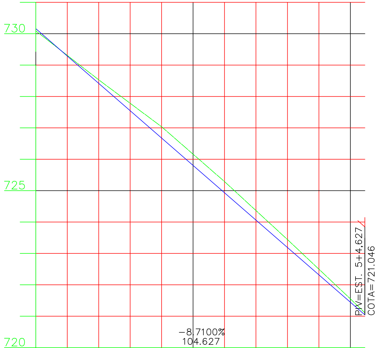
PERFIL RUA JOSE NOGUEIRO DOS SANTOS
