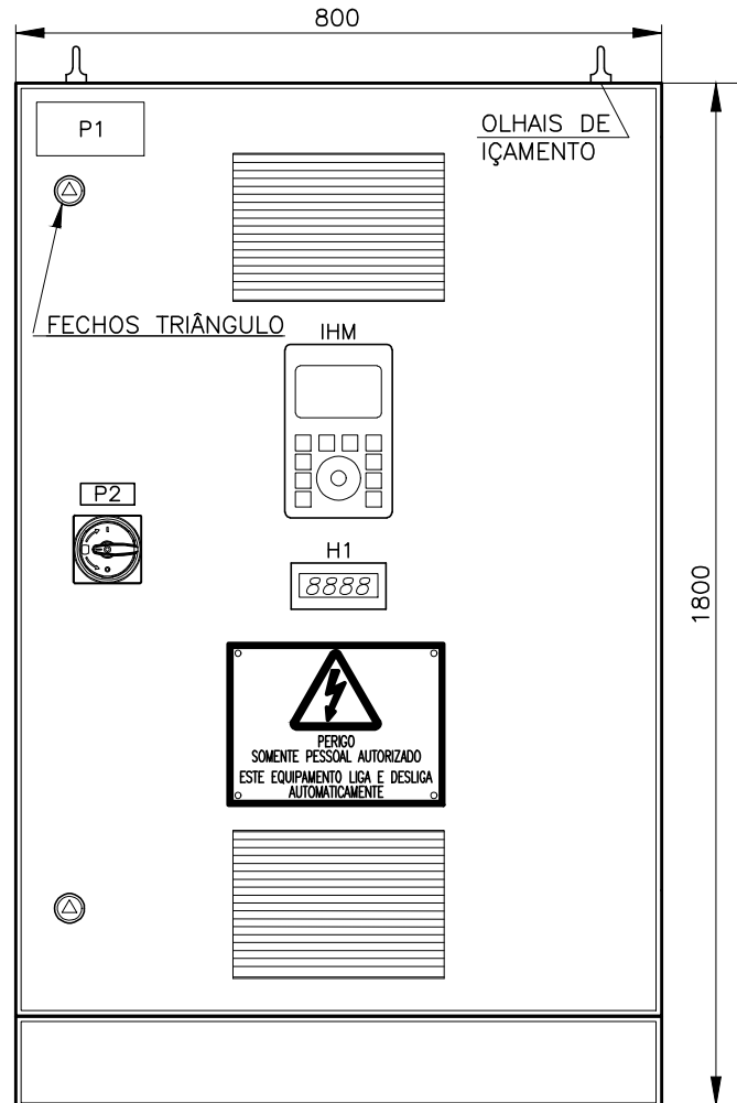
LAYOUT ORIENTATIVO
