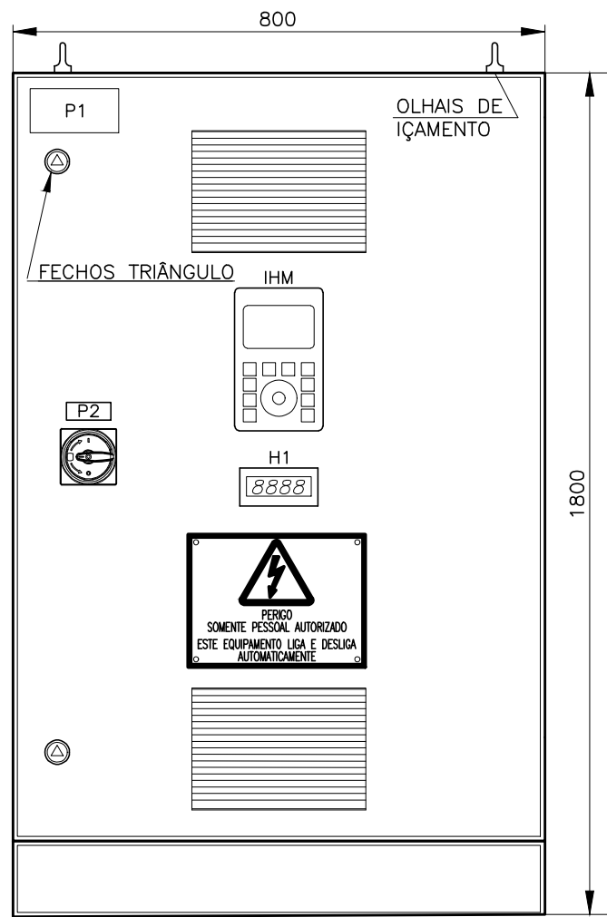
LAYOUT ORIENTATIVO
