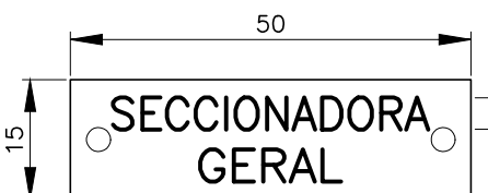
PLAQUETA 15X50 - ESC. 1:1
