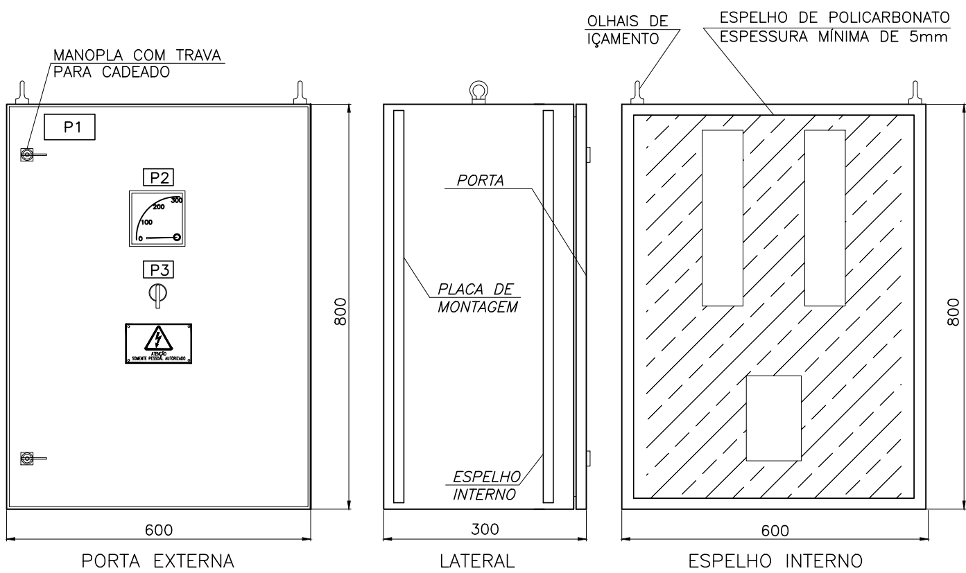
LAYOUT DO PAINEL SEM ESCALA
