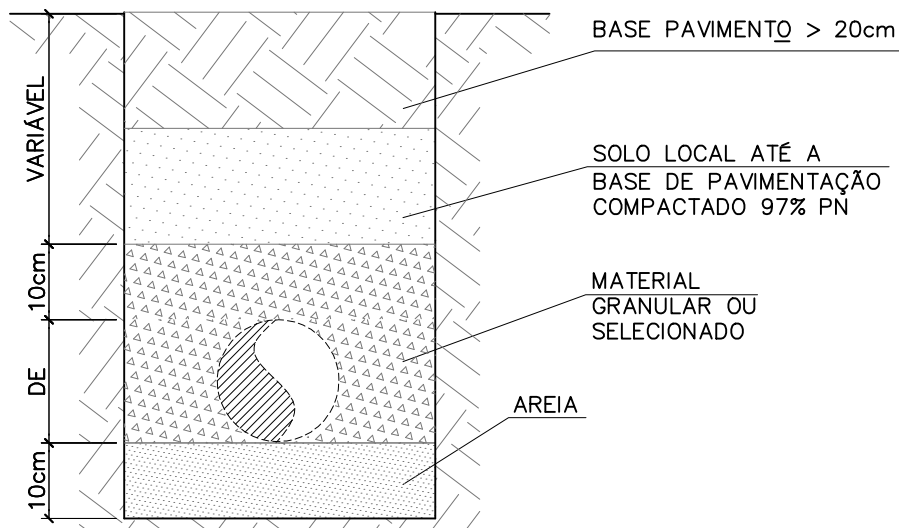
DETALHE-EMBASAMENTO DAS VALAS SEM ESC.
