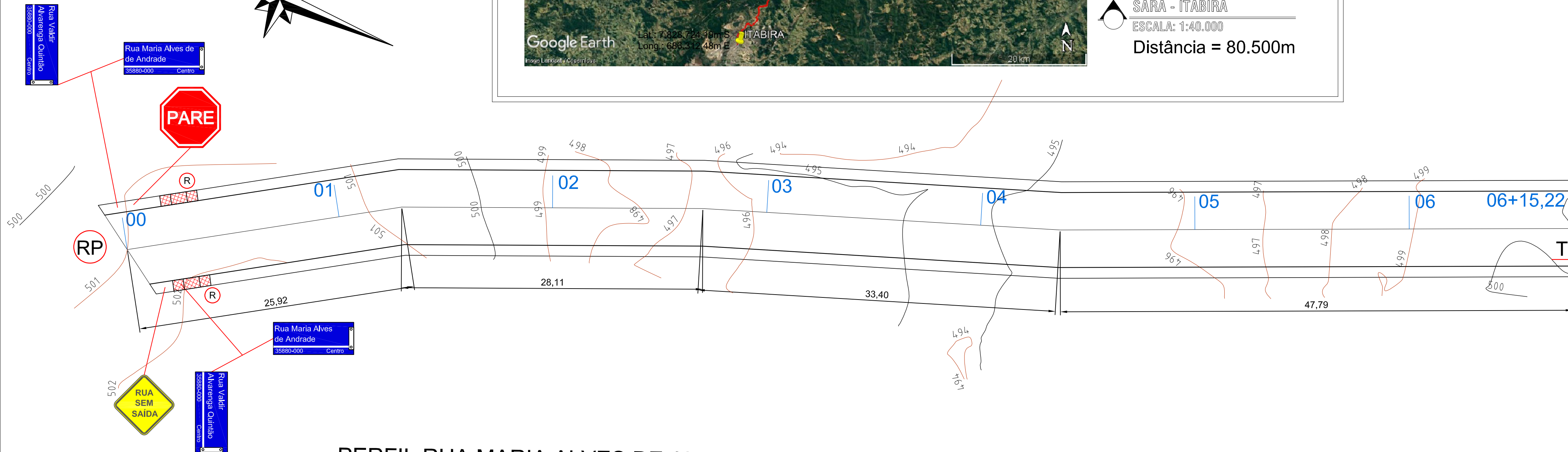
PERFIL RUA MARIA ALVES DE ANDRADE
