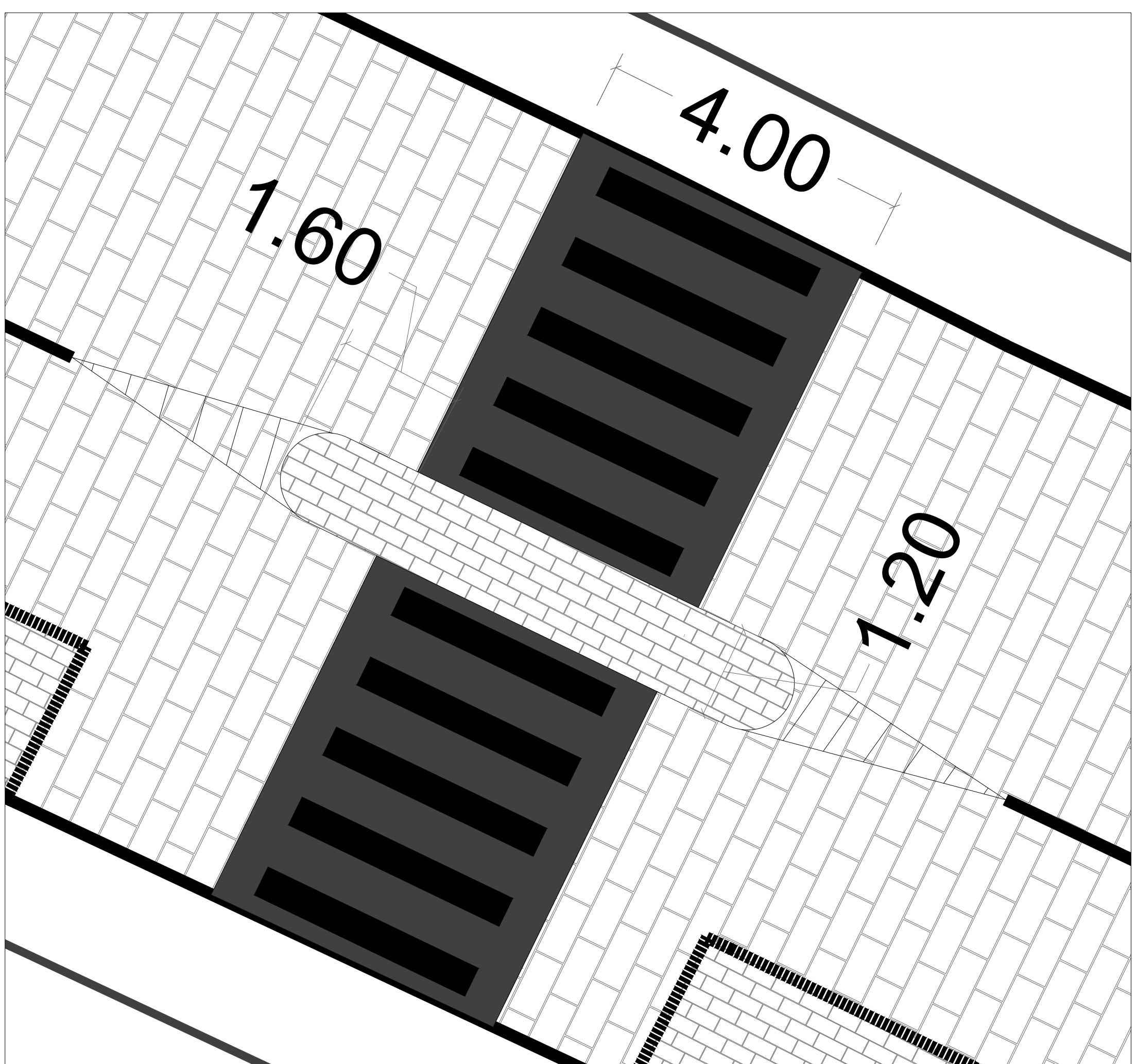
DETALHE DA PASSAGEM DE PEDESTRE ESC. 1:50
