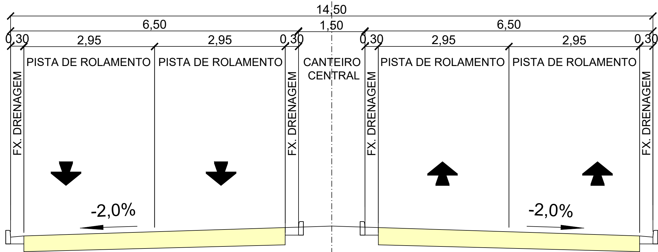
CORTE TRANSVERSAL ESC.: 1/50
