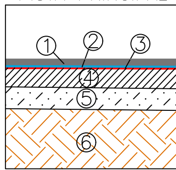
DETALHE 1 – PAVIMENTO NOVO PISTA PRINCIPAL
