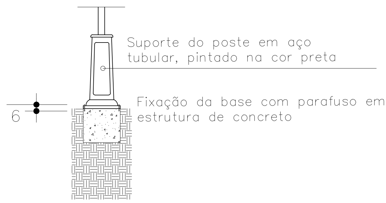
DET.5 – BASE POSTE JARDIM ESCALA 1/20
