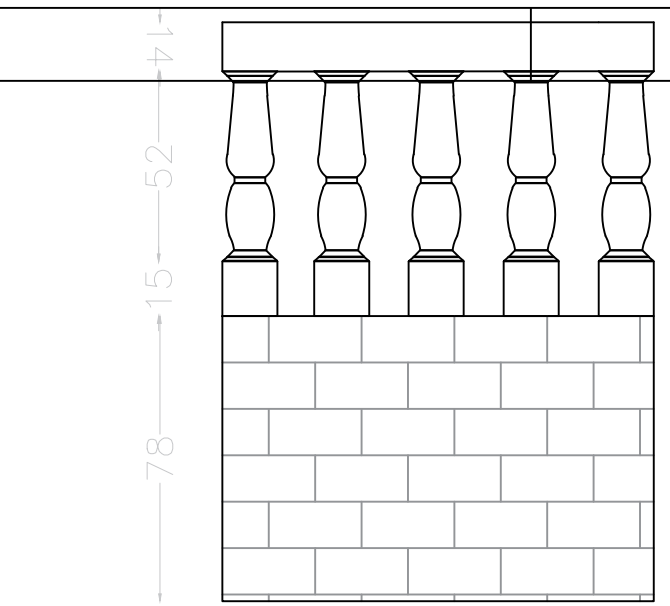
DET.1 – BALAUSTRE ESCALA 1/20
