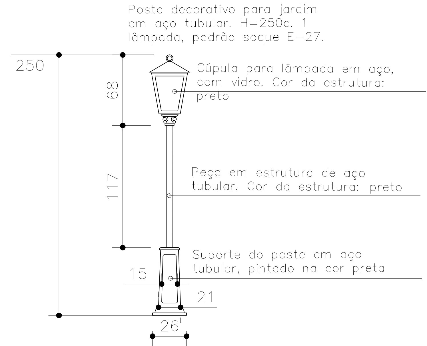
DET.3 – POSTE JARDIM ESCALA 1/20
