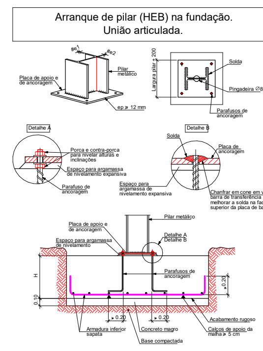
Det. Arranque de Poste 1 : 50
