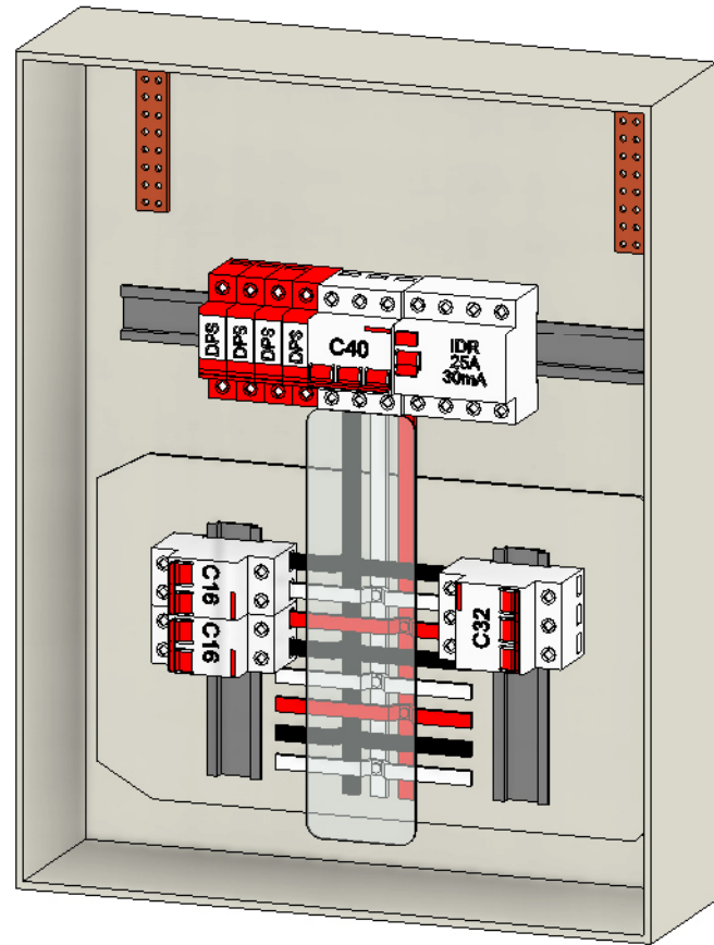
Det. Quadro de Distribuição de Circuitos
