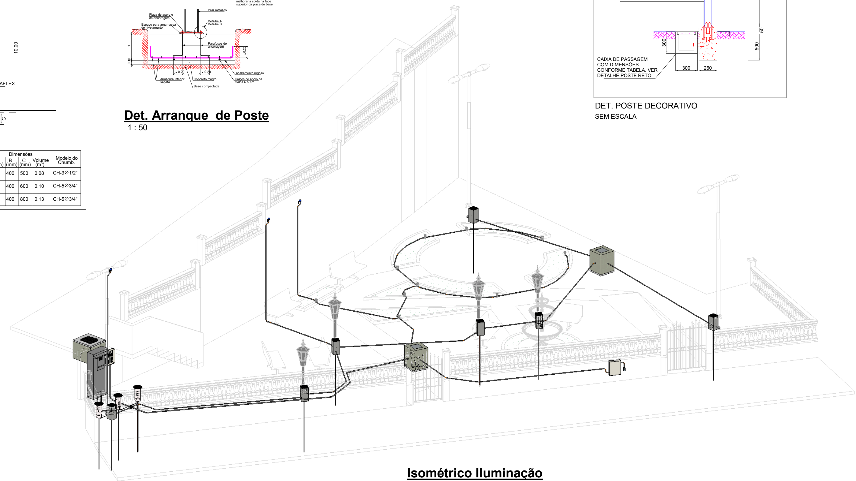
Isométrico Iluminação
