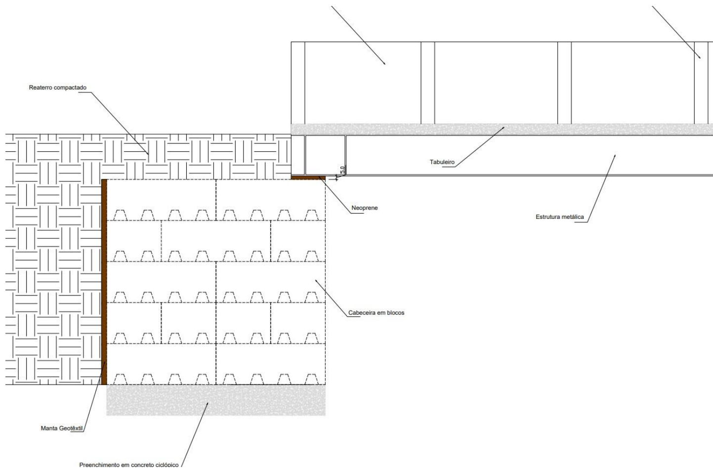
Figura 02: cabeceira projetada com blocos pré-moldados.
