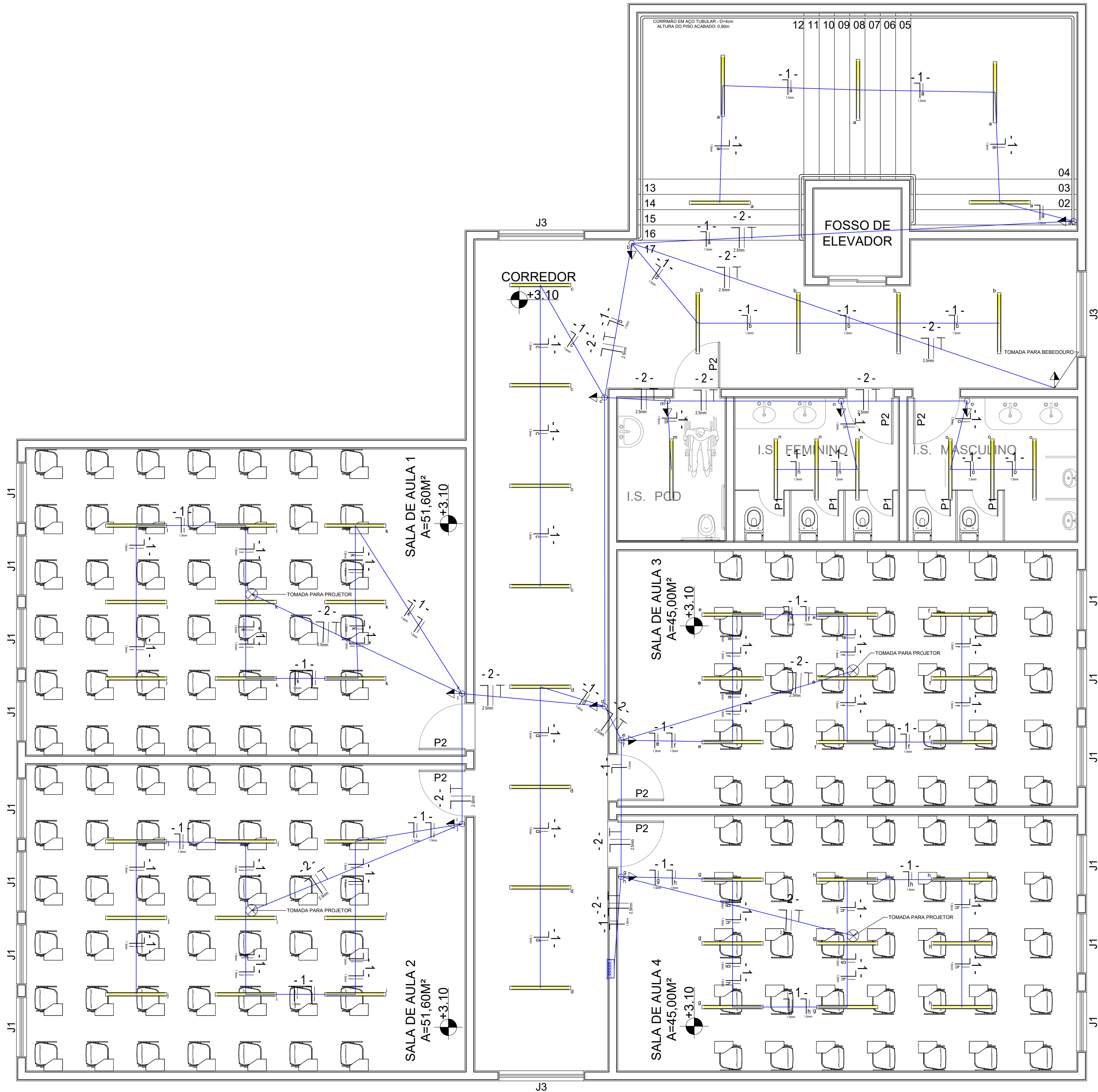
PLANTA SEGUNDO PAVIMENTO ESCALA 1:50
