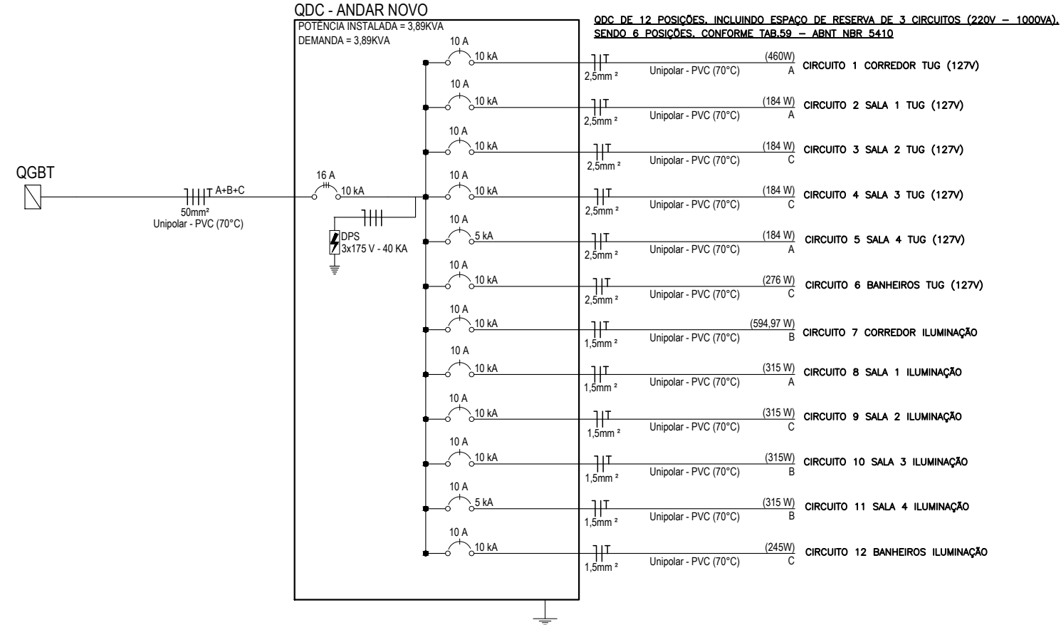
DIAGRAMA UNIFILAR SEM ESCALA
