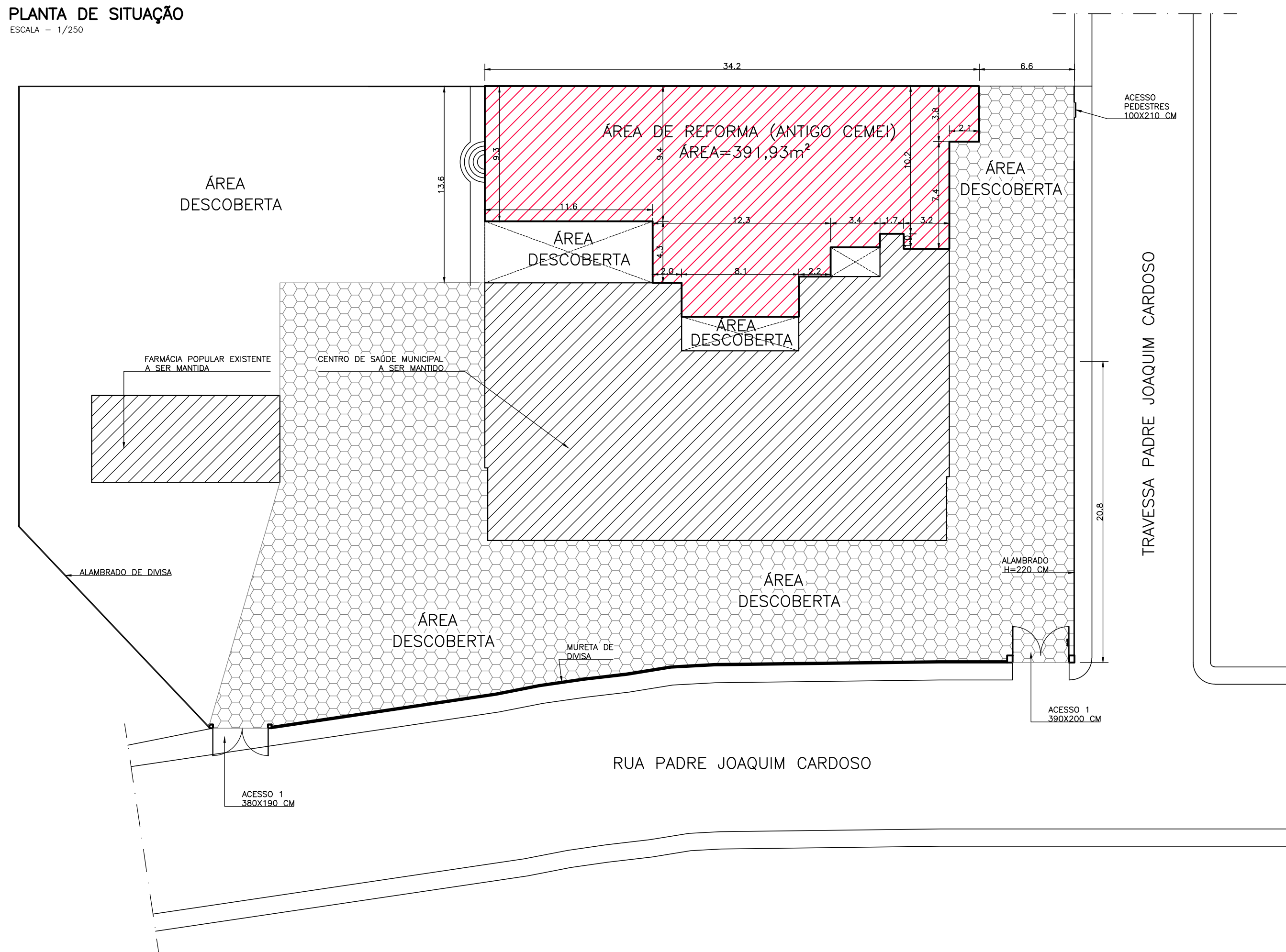
PLANTA DE SITUAÇÃO ESCALA - 1/200
