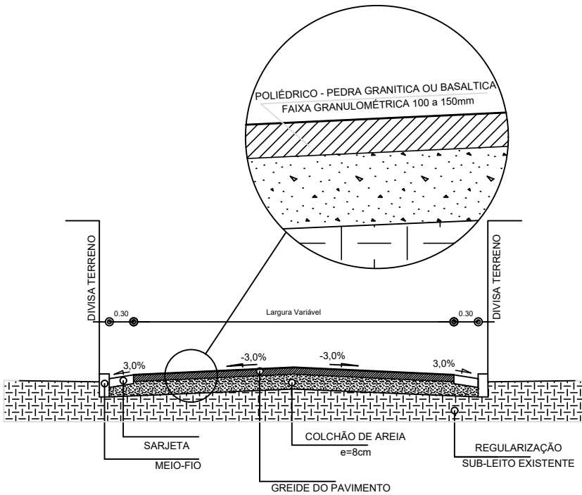
DETALHAMENTO DE SARJETA E MEIO-FIO DE CONCRETO DESENHO REPRESENTATIVO - SEM ESCALA
