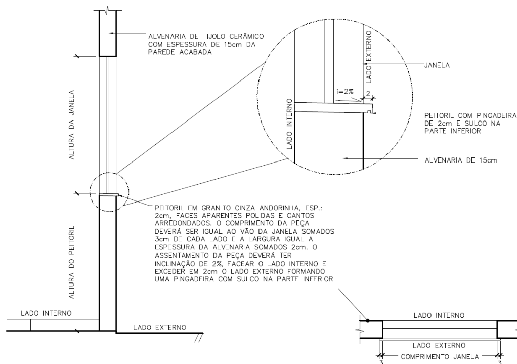
DETALHE 4 ESCALA 1:20 TÍPICO PINGADEIRA
