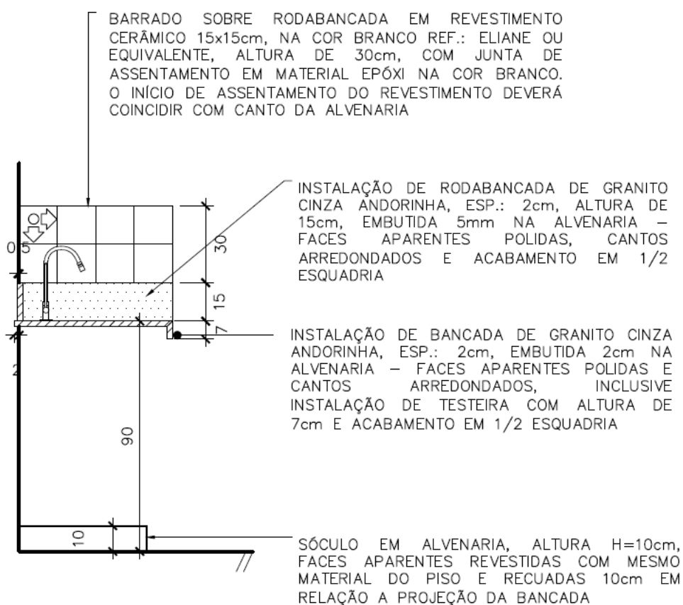
DETALHE 2 ESCALA 1:20 TÍPICO BANCADA SECA
