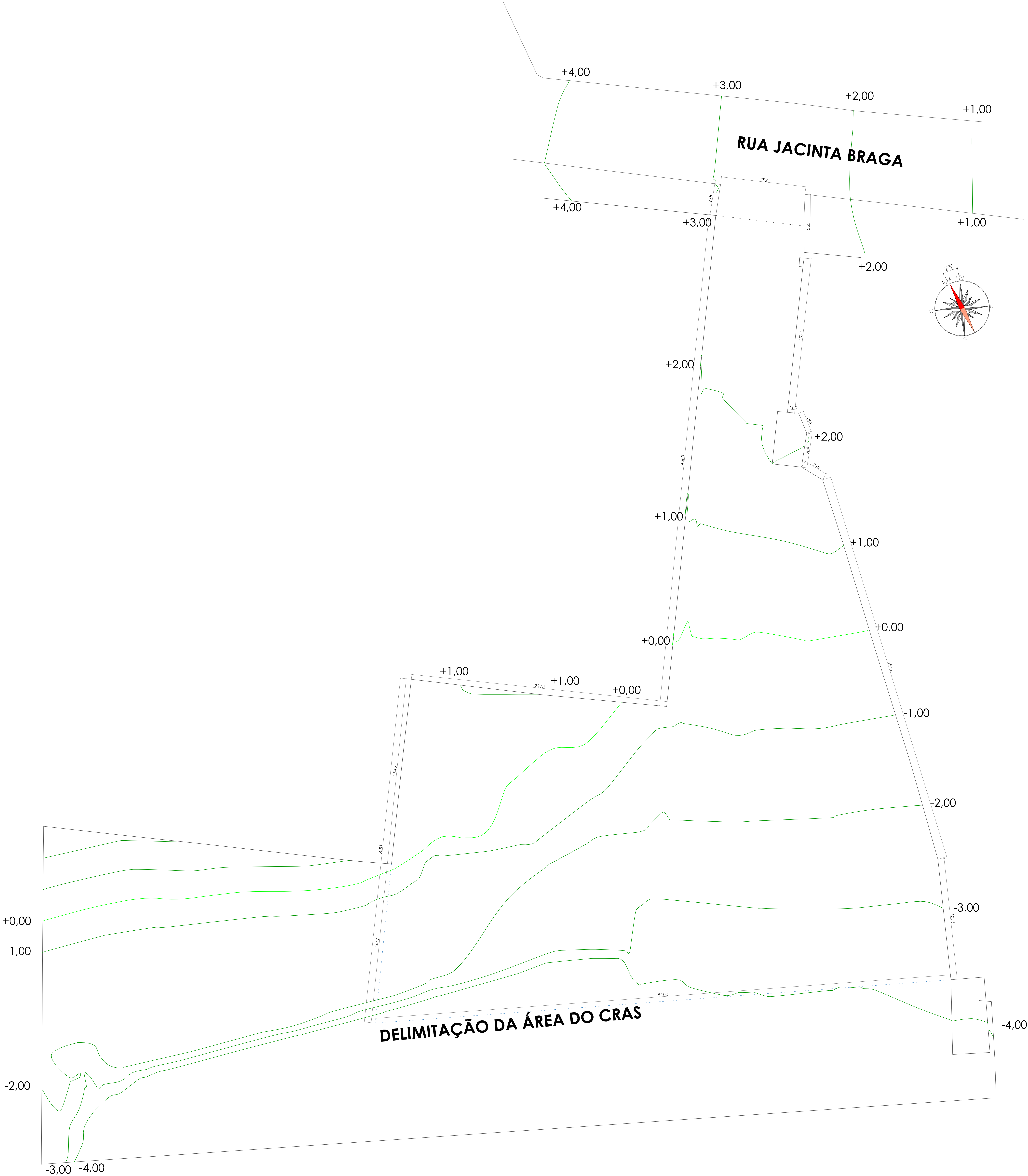
PLANTA BAIXA LEVANTAMENTO PLANIALTIMÉTRICO ÁREA: 3.185,59m² ESC. (A0): 1 | 100
