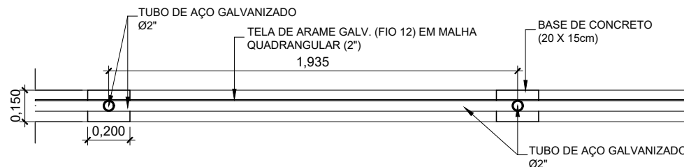
3 PLANTA - ALAMBRADO 1:25
