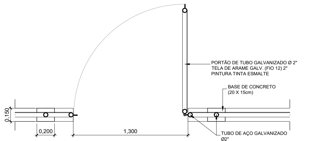
1 PLANTA - PORTÃO SIMPLES 1:25
