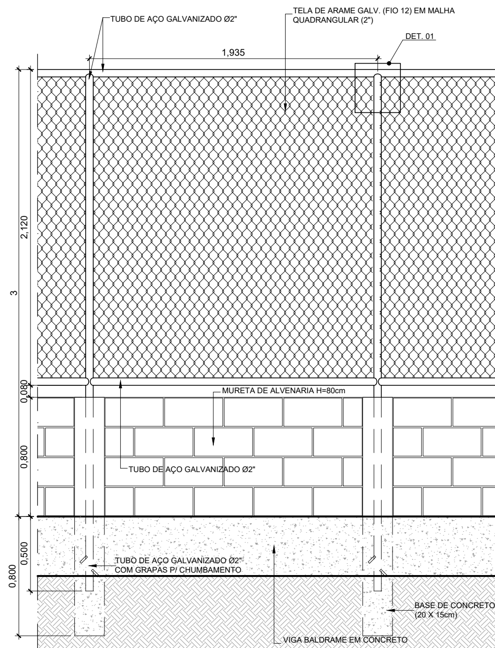
4 VISTA - ALAMBRADO 1:25
