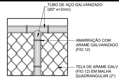
6 DETALHE 1 - ALAMBRADO 1:10
