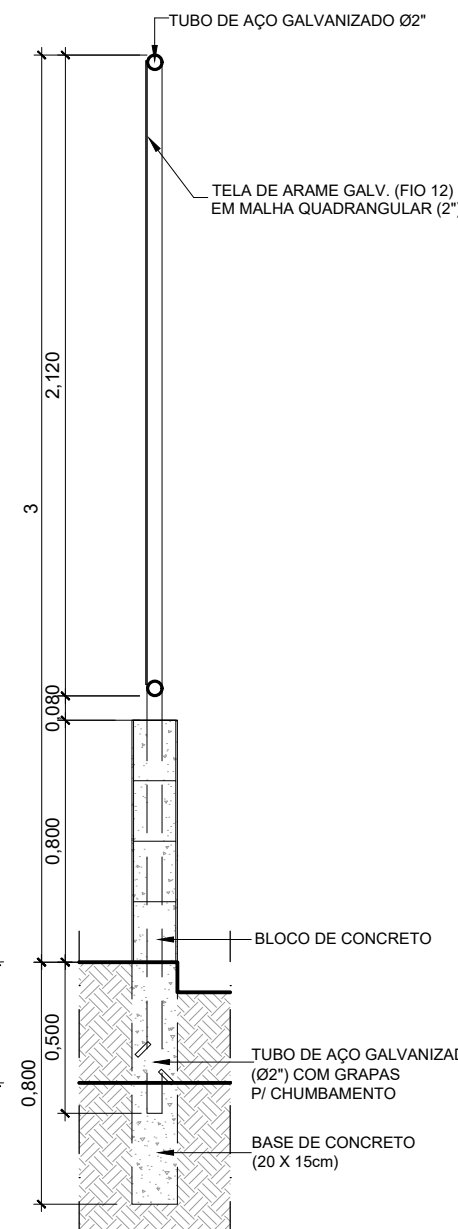
5 CORTE - ALAMBRADO 1:25
