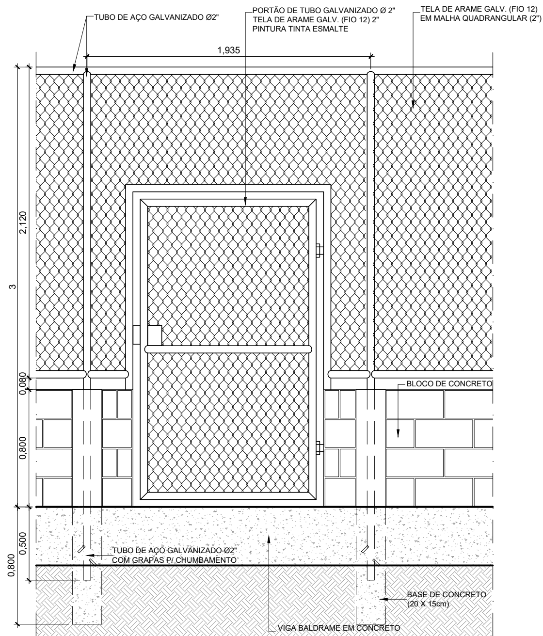
2 VISTA - PORTÃO SIMPES 1:25
