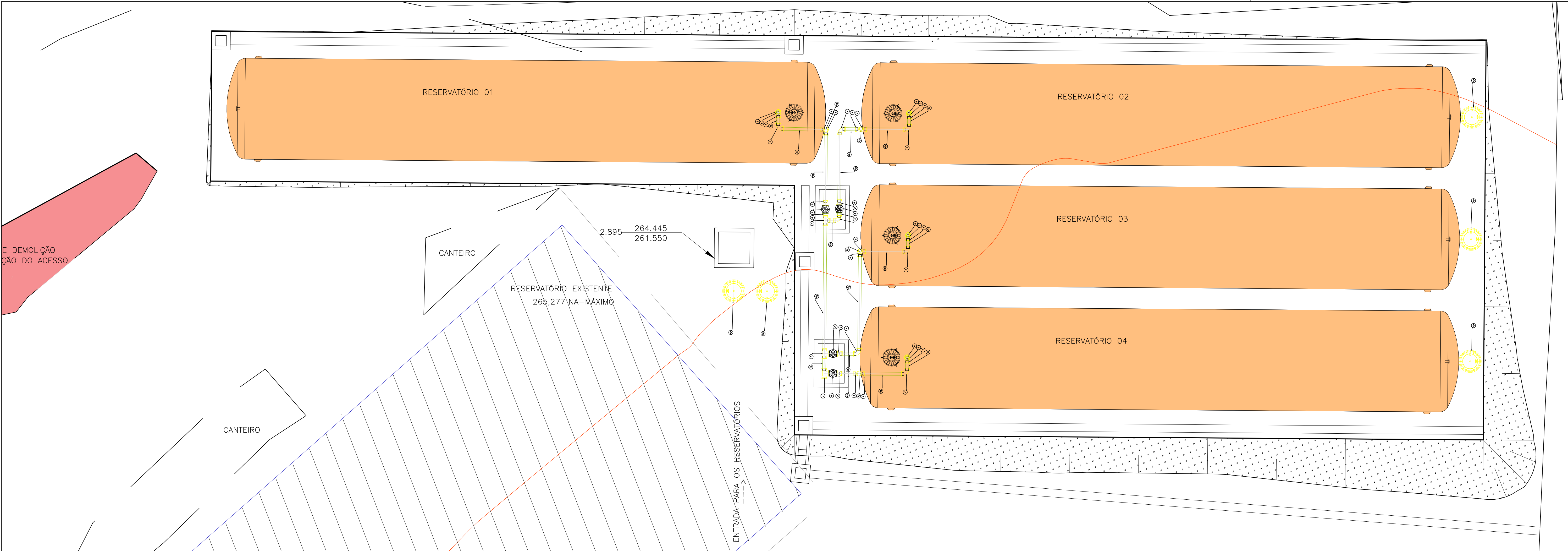
ALIMENTAÇÃO DOS RESERVATÓRIOS ESC. 1:75
