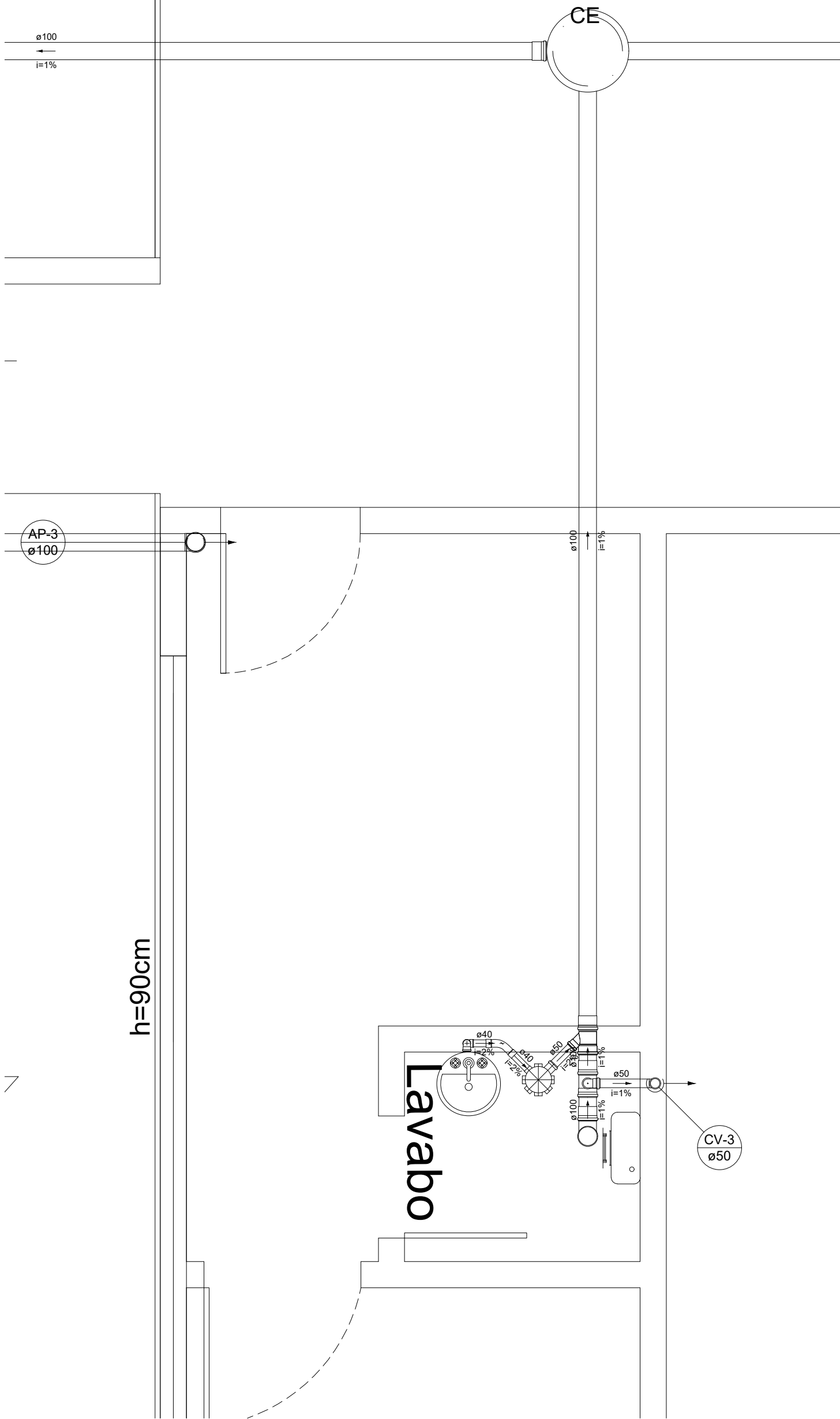
Detalhe S2 Escala 1:25
