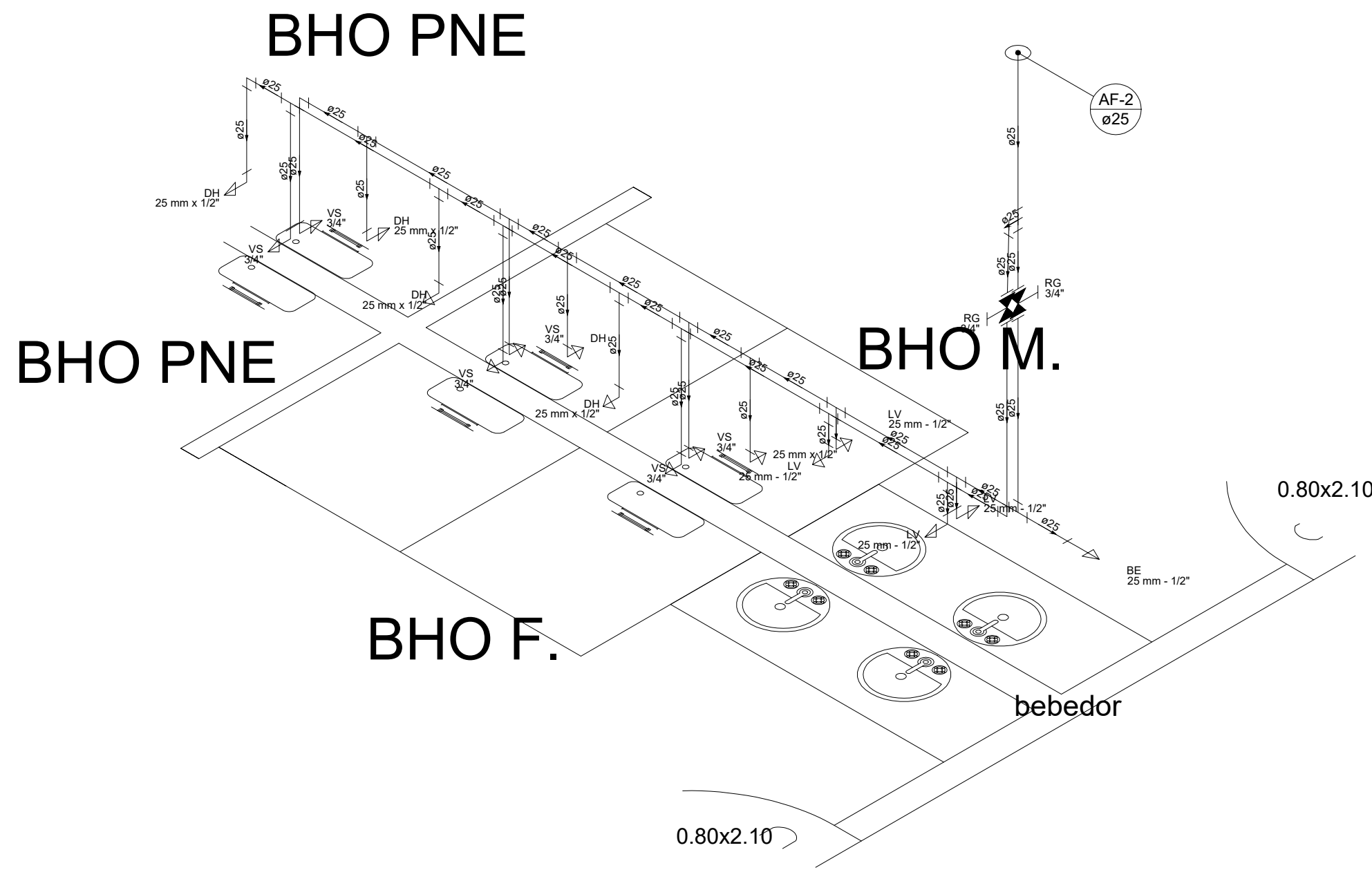
Detalhe H4 Escala 1:25
