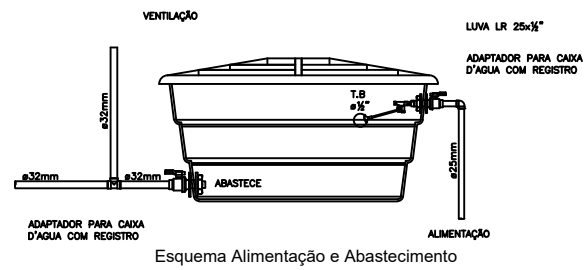
Detalhe Ligação de Caixa d'água Polietileno Sem Escala
