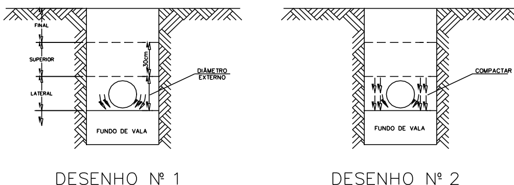
Figura 7 - Detalhes de Reaterro de Vala
