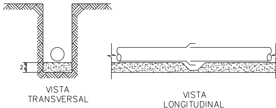
Figura 5 – Em solo rochoso sem a presença de água.
