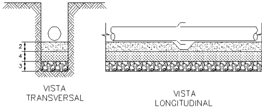
Figura 4 - Em solo que não oferece condições mecânicas de suporte, com presença de água.
