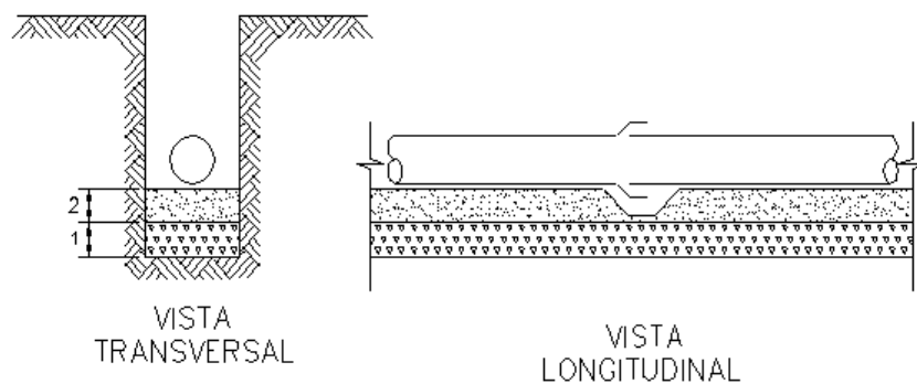
Figura 2 - Normal com normal com presença de água: quando o solo oferece condições mecânicas de suporte, porém, com presença de água.
