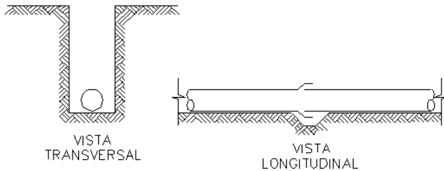
Figura 1 – Normal, quando o solo oferece condições mecânicas de suporte e é isento de pedras ou objetos duros
