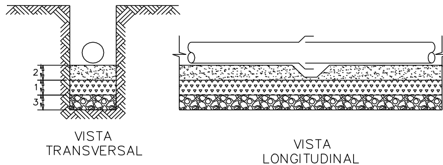
Figura 5 – Em solo rochoso sem a presença de água.
