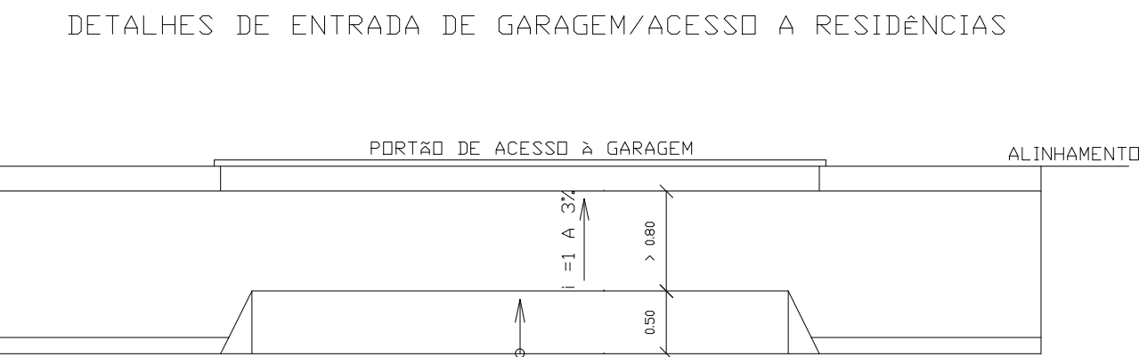
DETALHE ENTRADA DE GARAGEM SEM ESCALA
