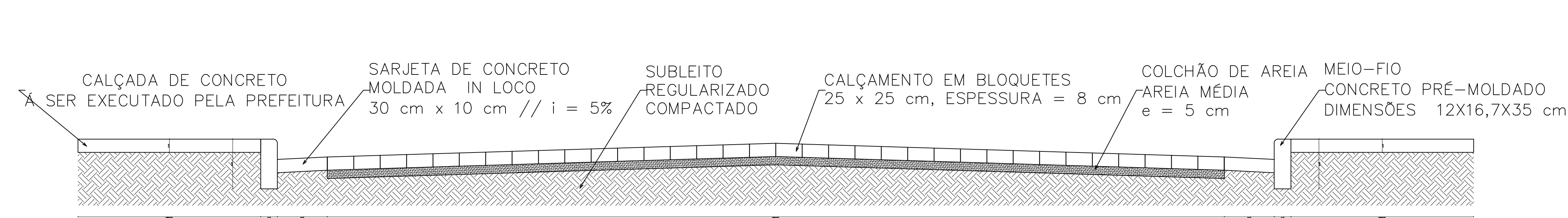
CORTE TRANSVERSAL
