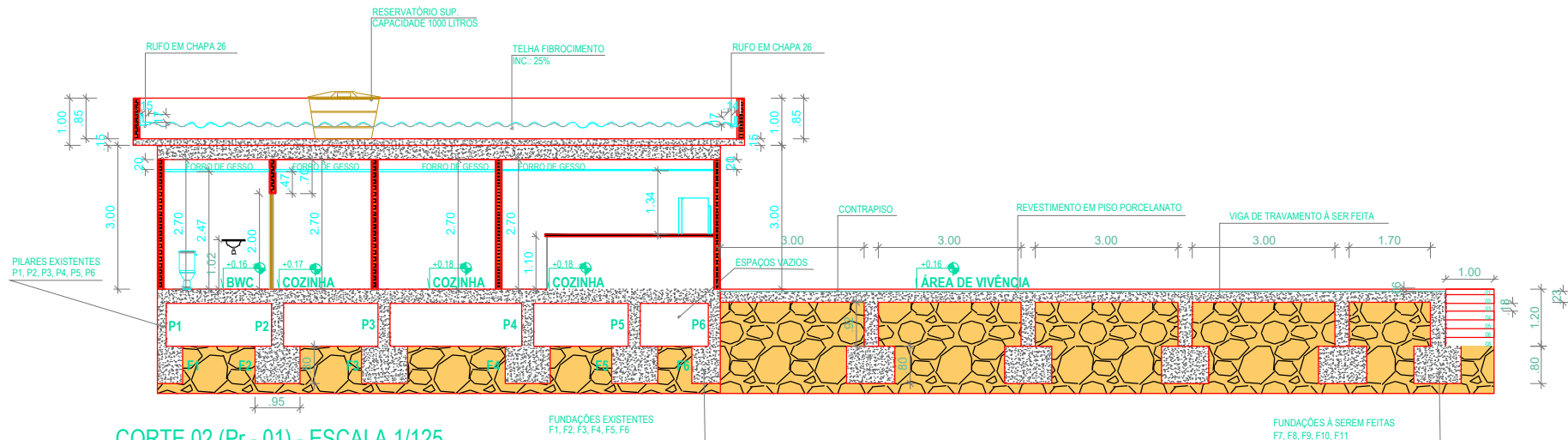
CORTE 02 (Pr - 01) - ESCALA 1/125
