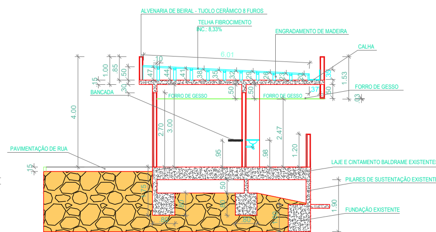
CORTE 01 (Pr - 01) - ESCALA 1/125
