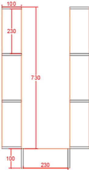
PLANTA BAIXA
