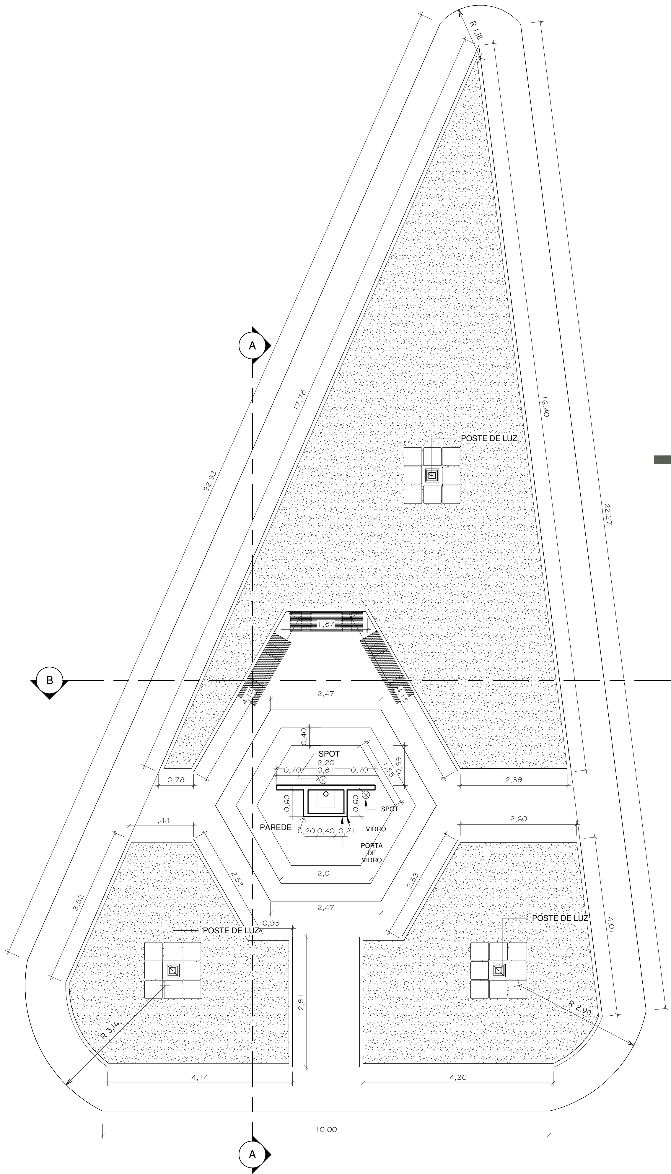
1 PLANTA BAIXA 1 : 50
