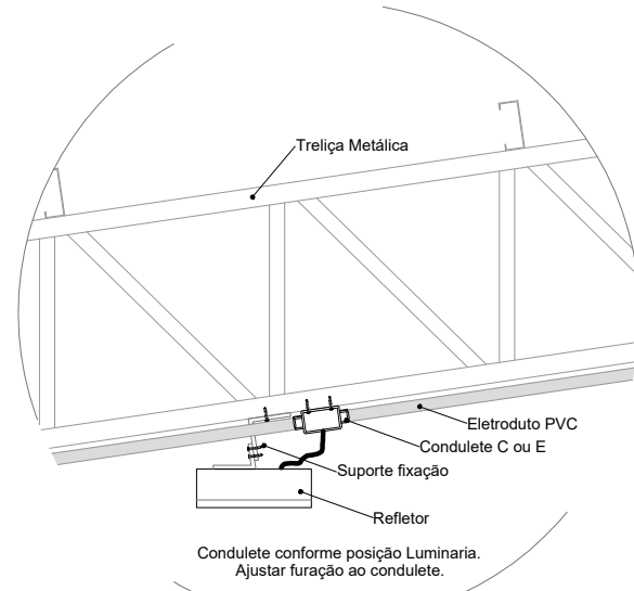
3 DETALHE FIXAÇÃO DO REFLETOR ESCALA: SEM
