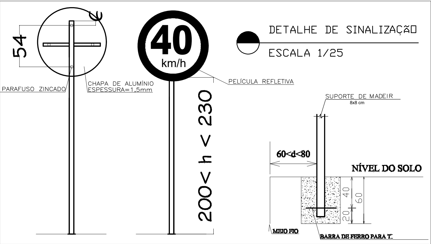
DETALHE SINALIZAÇÃO PLACA DE VELOCIDADE E PARE ESCALA 1/25
