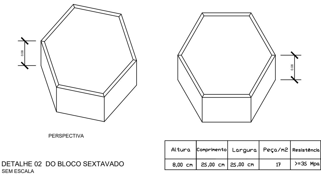
Detalhe 02
