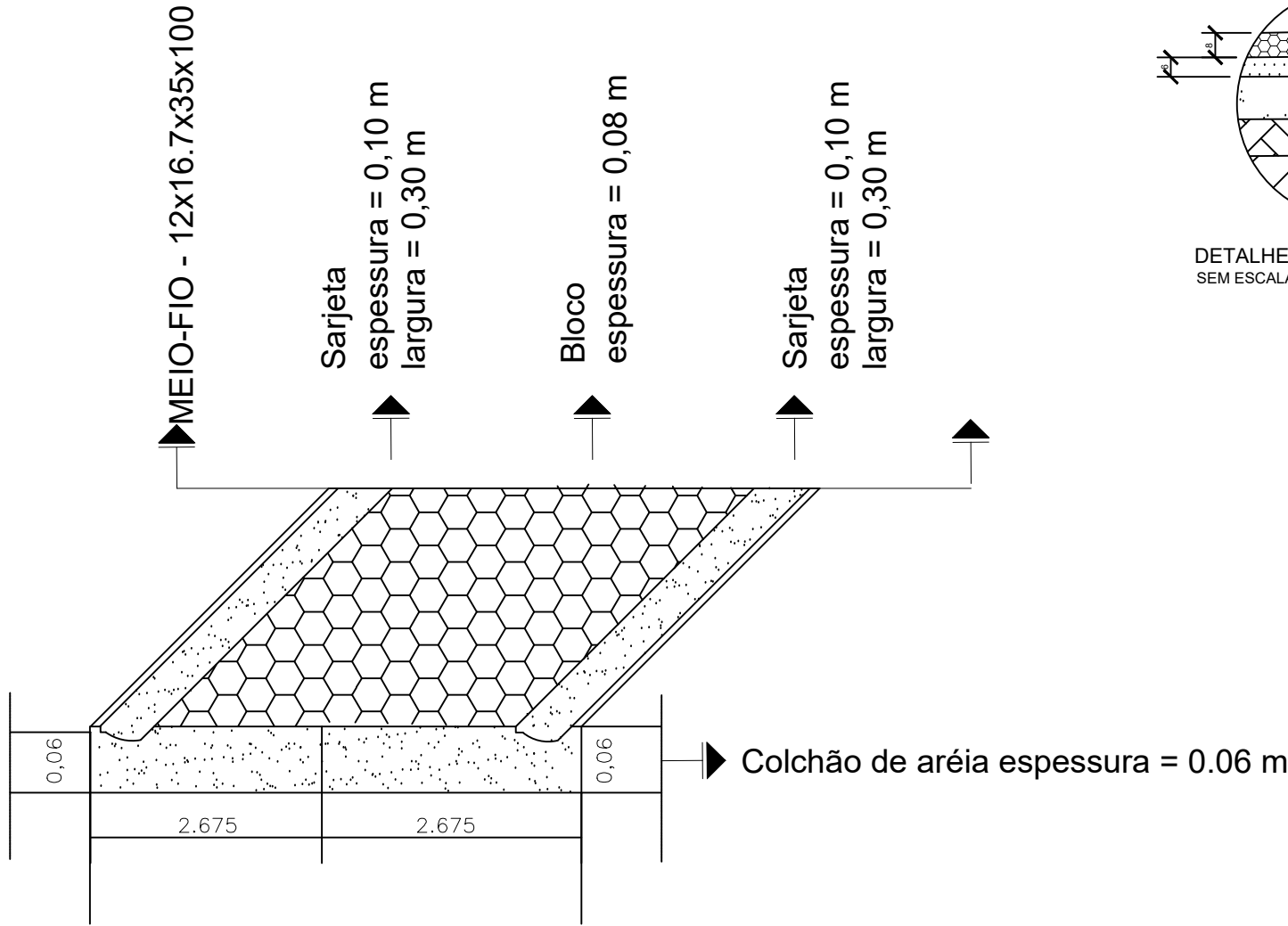
DETALHE DO CALÇAMENTO DE RUAS SEM ESCALA
