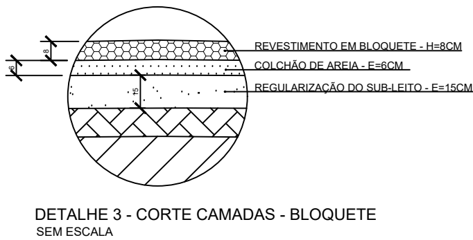
Detalhe 03
