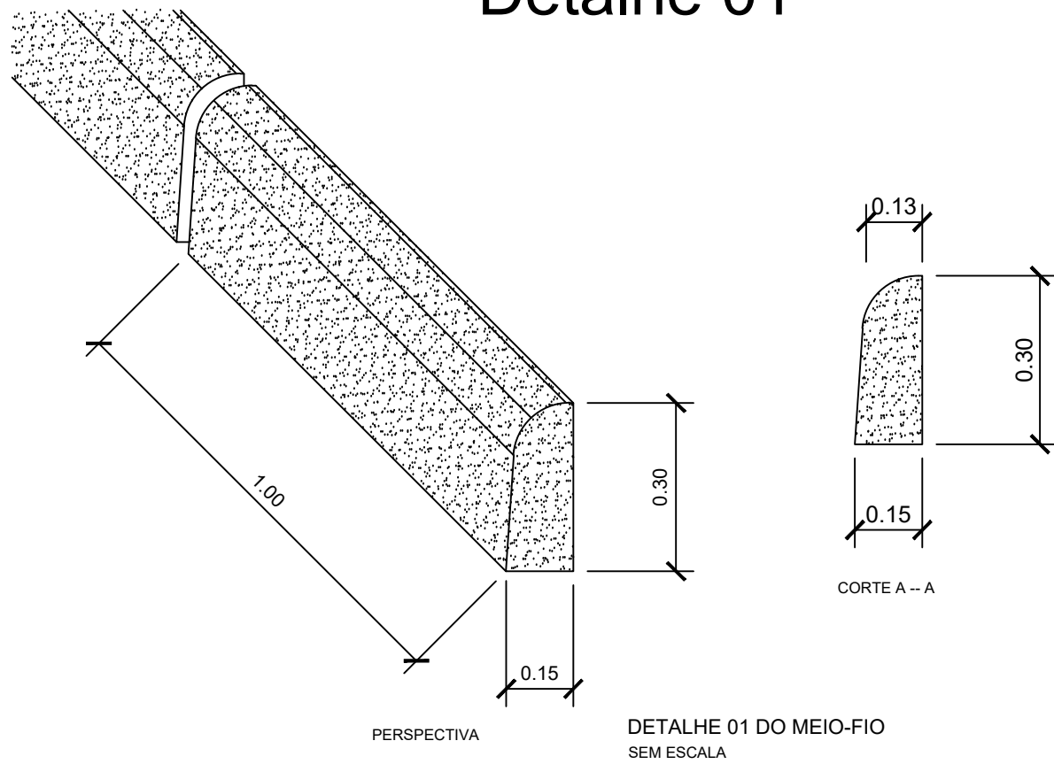
Detalhe 01
