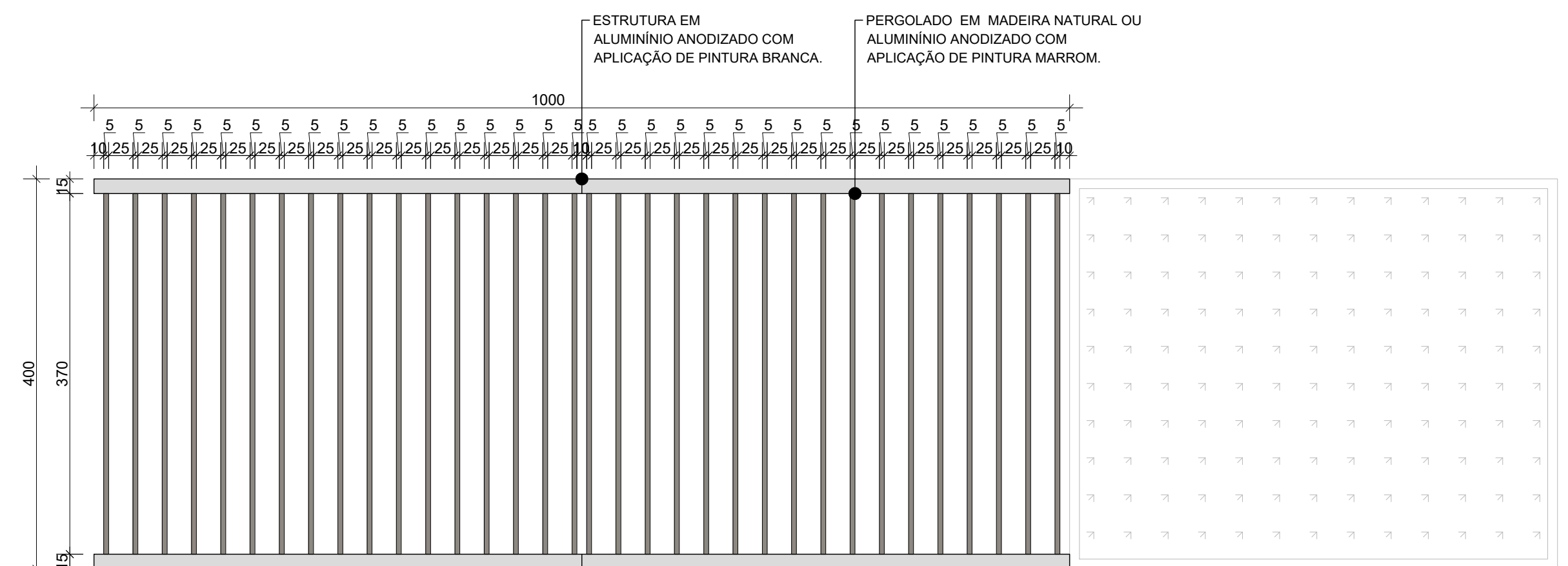
7 PLANTA DE COBERTURA - MÓDULO PERGOLADO
