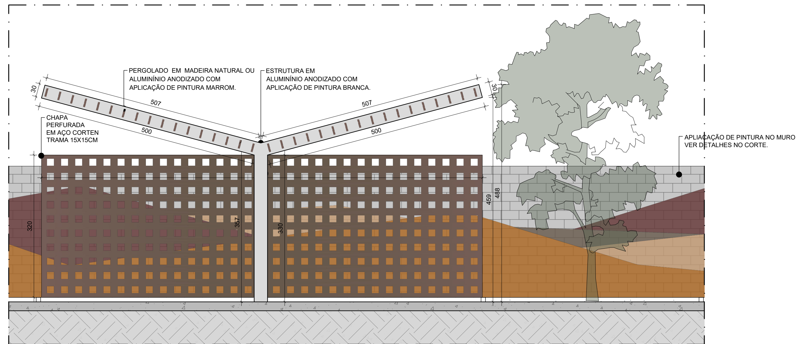
11 CORTE - MÓDULO PERGOLADO
