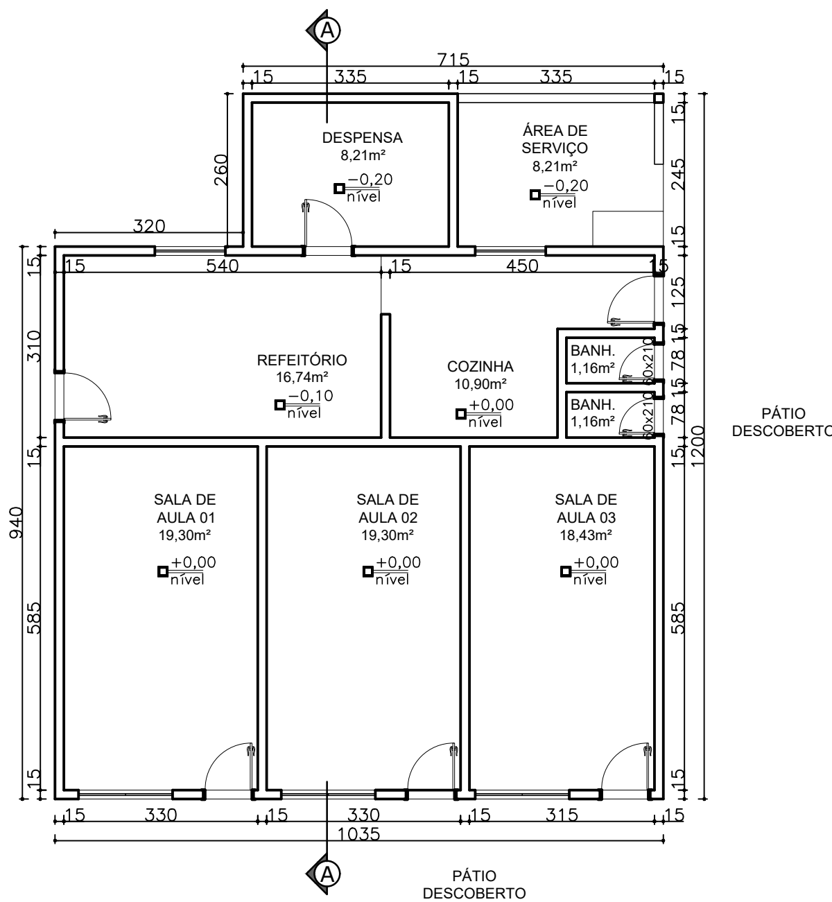
ESCOLA EXISTENTE A SER DEMOLIDA ESC:1/100
