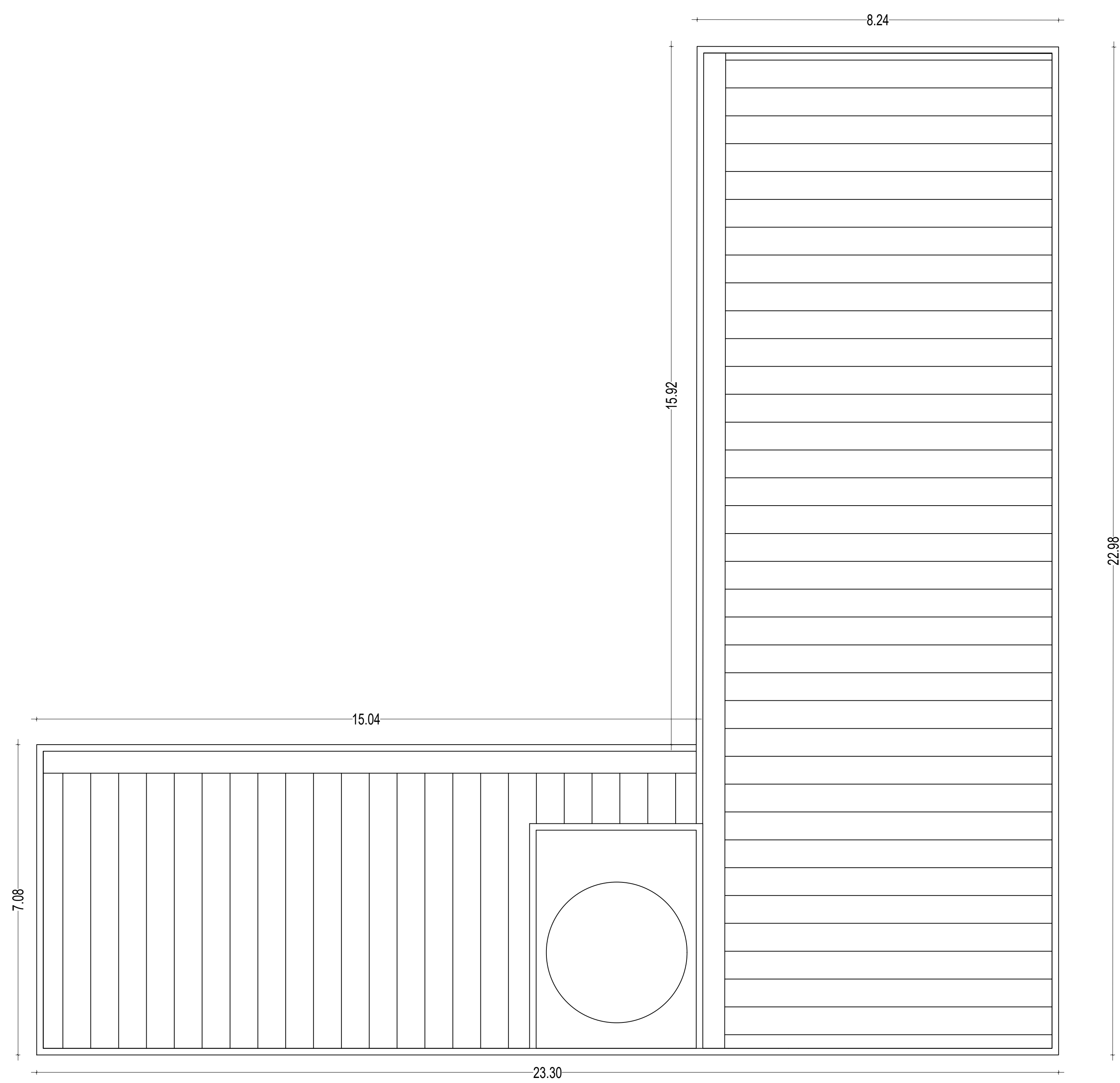
PLANTA DE COBERTURA ESC:1/75
