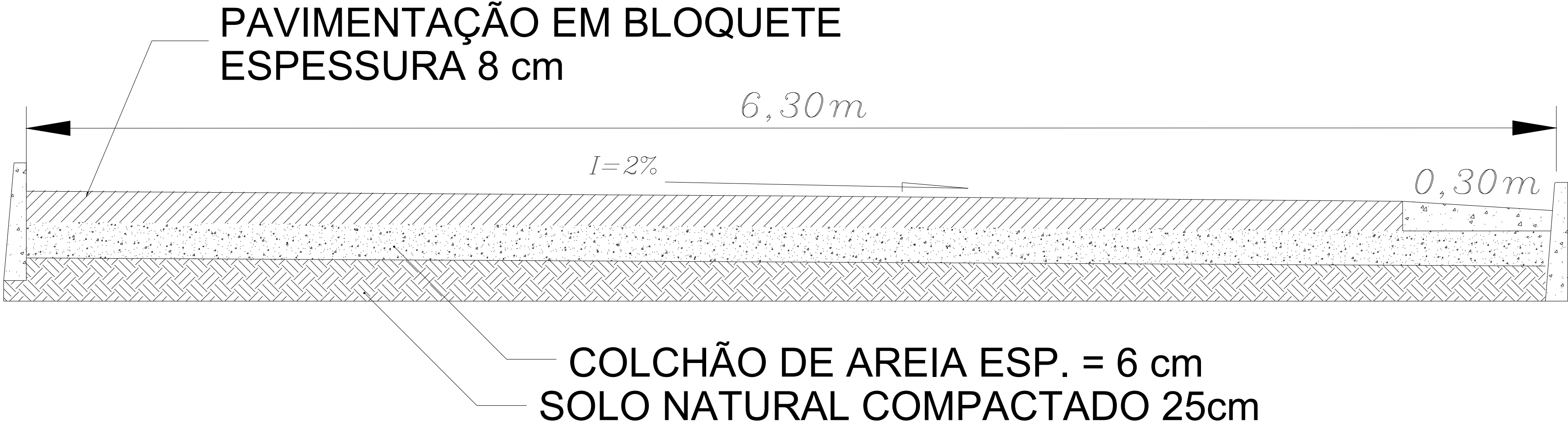
SEÇÃO TRANSVERSAL SEM ESCALA
