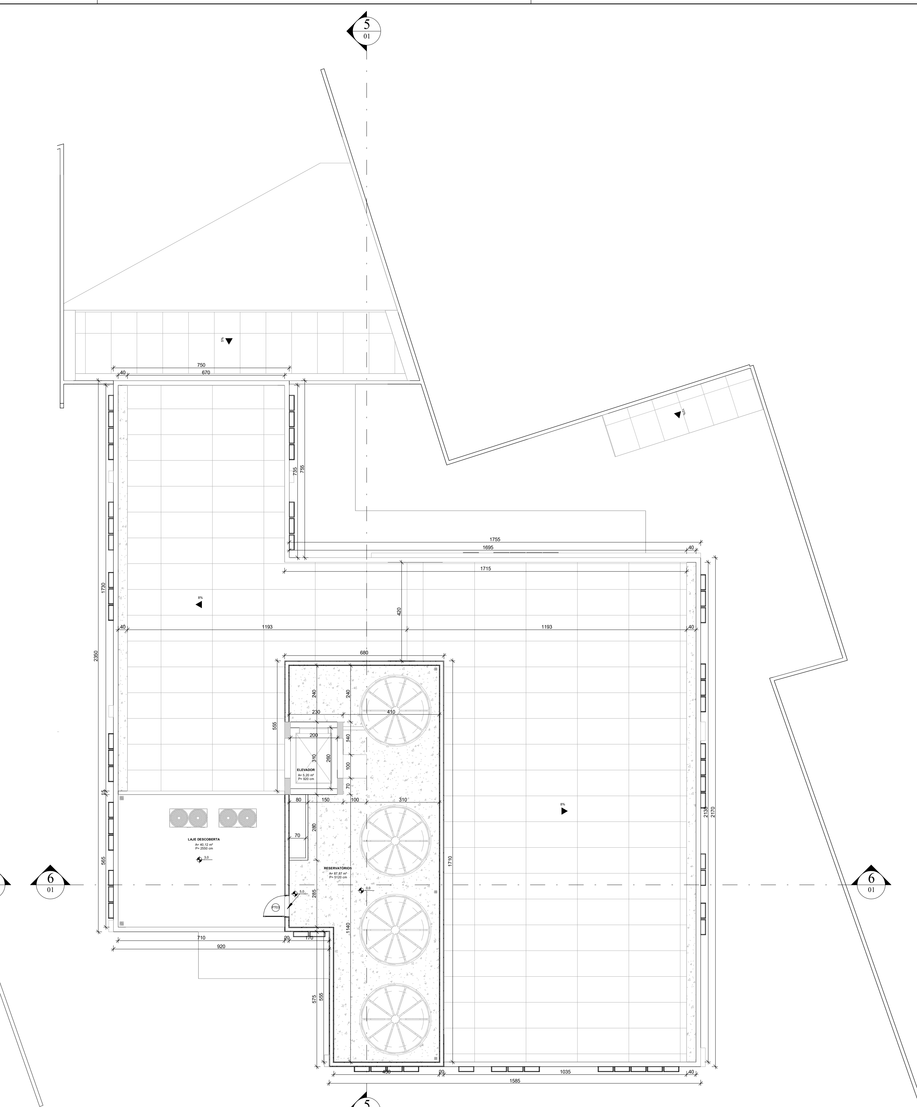
3 HM-NV 03 1 : 100
