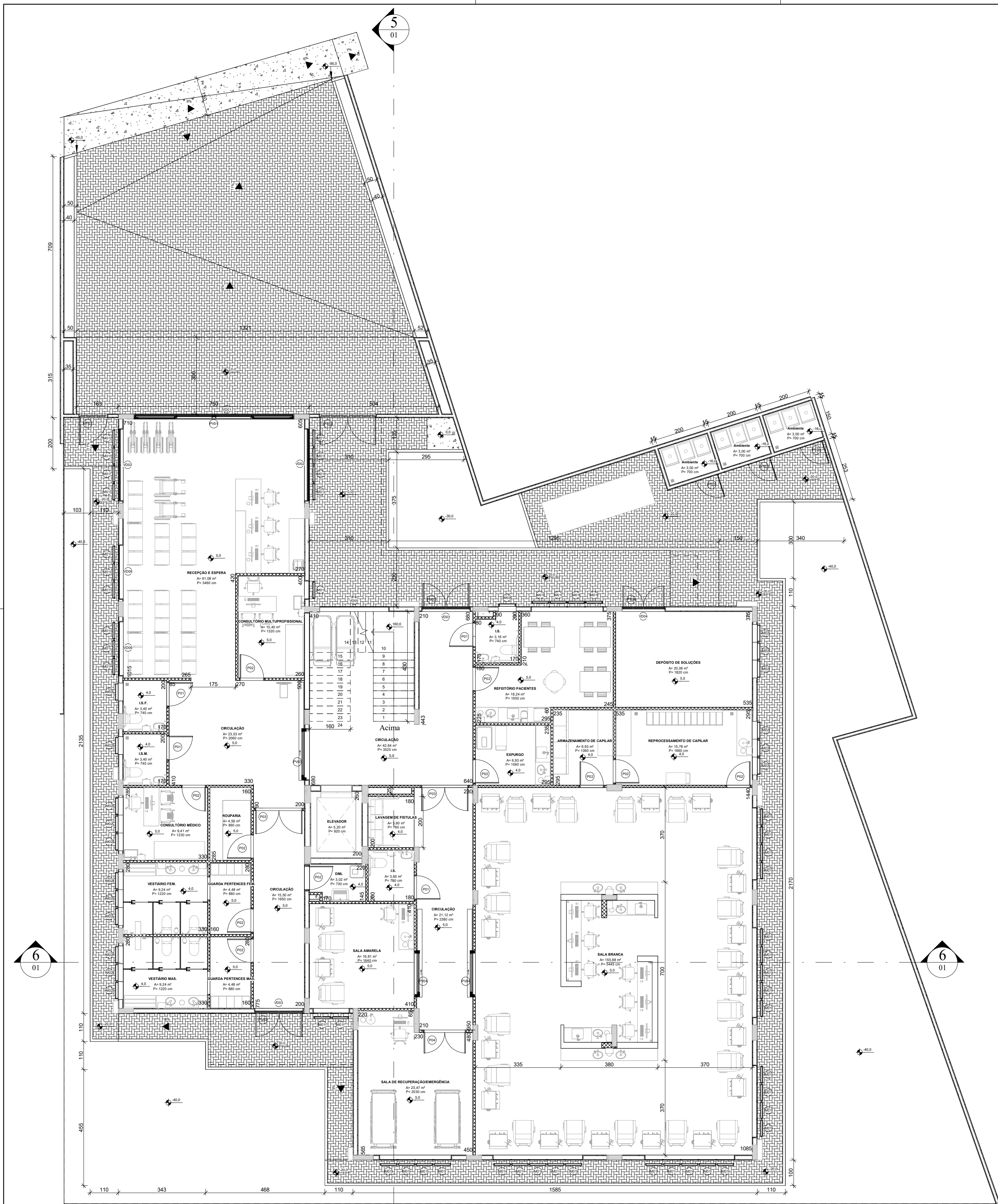
2 HM-NV 01 - PLANTA BAIXA 1 : 100
