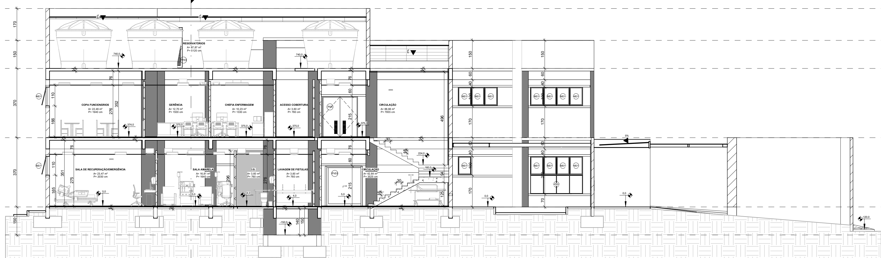
5 CORTE A-A 1 : 100
