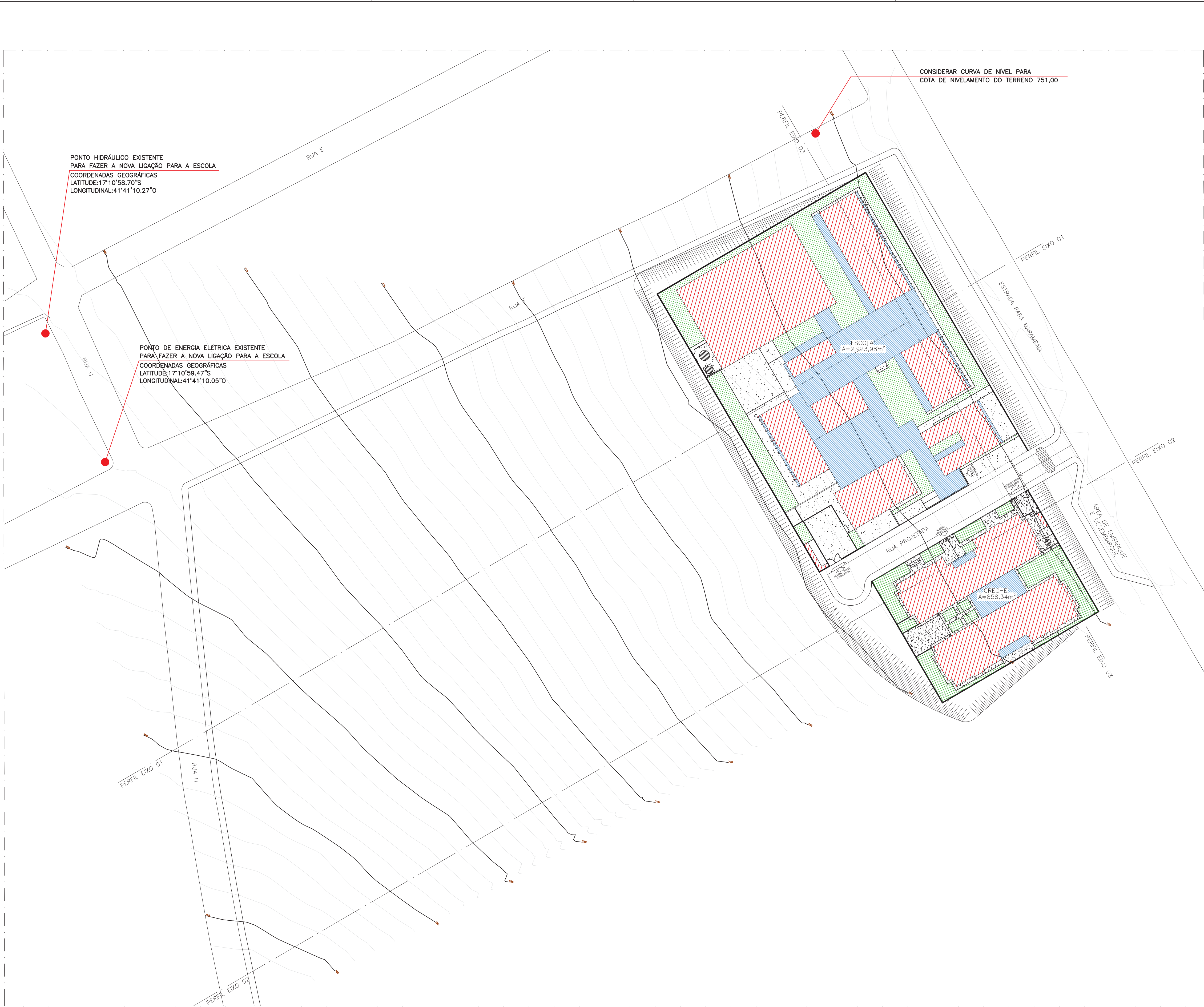
IMPLANTAÇÃO ESCALA 1:500
