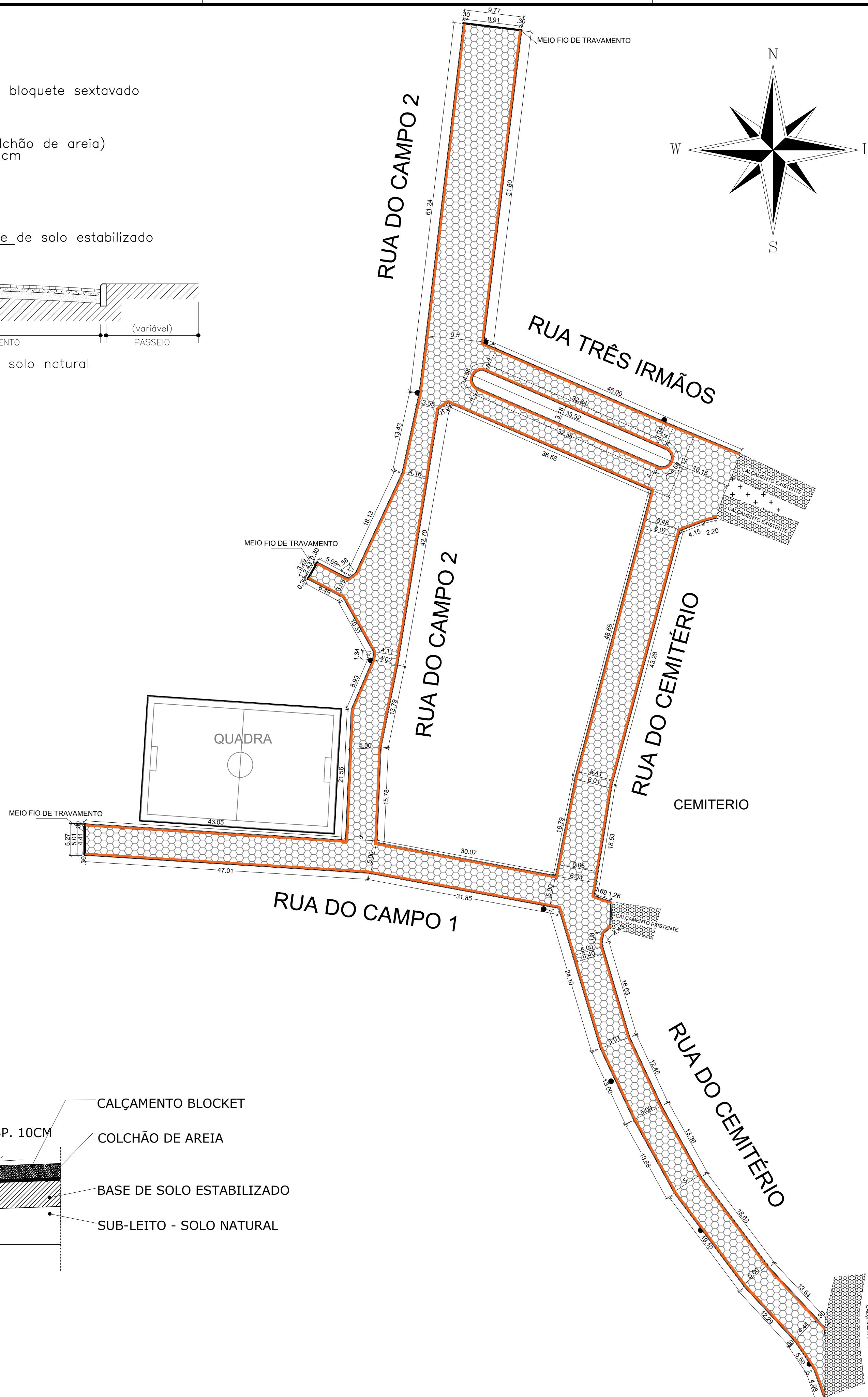
PLANTA DE PAVIMENTAÇÃO 1:400
