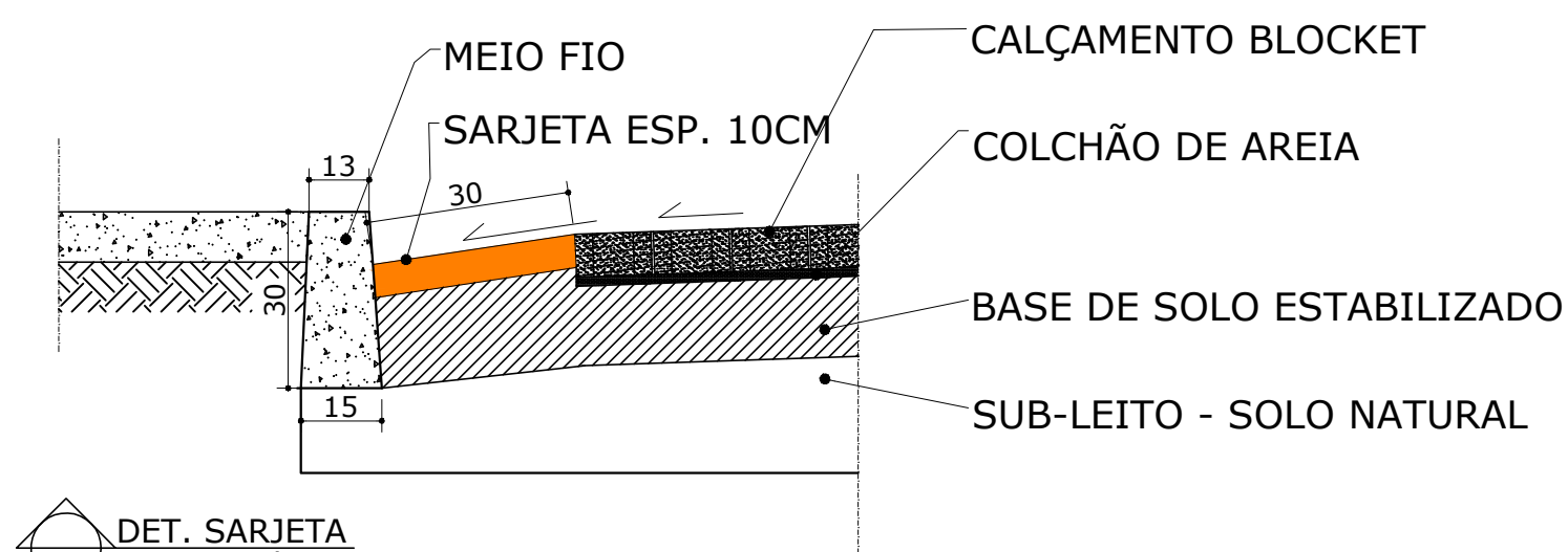
DET. SARJETA Sem escala
