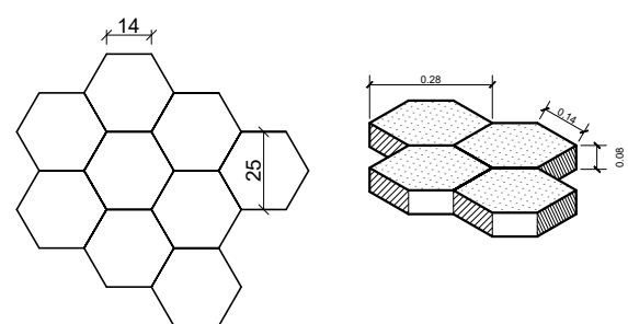
DETALHE DOS BLOCOS Sem escala
