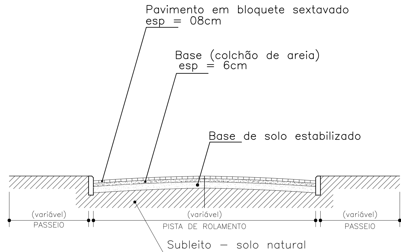
PERFIL TRANSVERSAL Sem escala
