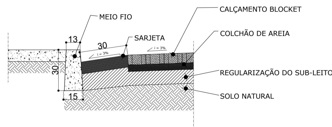
DET. SARJETA Sem escala
