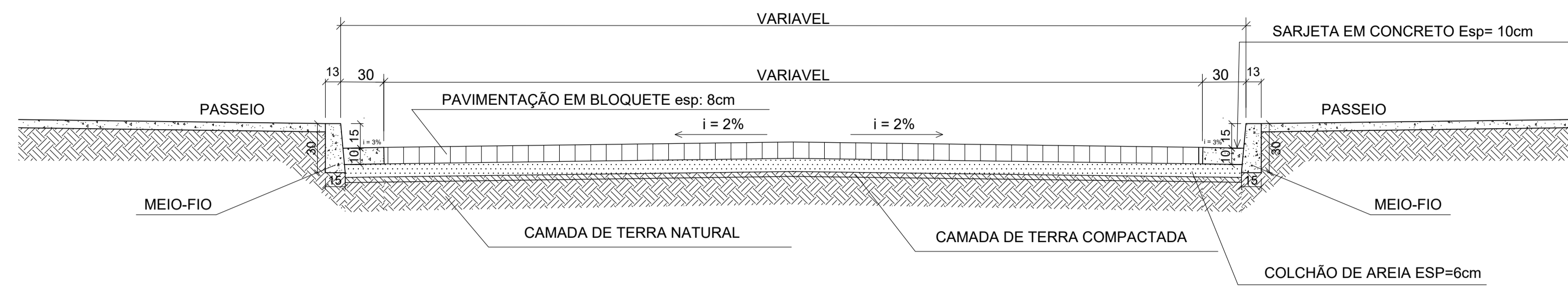
PERFIL TRANSVERSAL Sem escala
