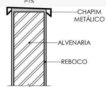
DETALHE - CHAPIM METÁLICO Escala: 1 : 10
