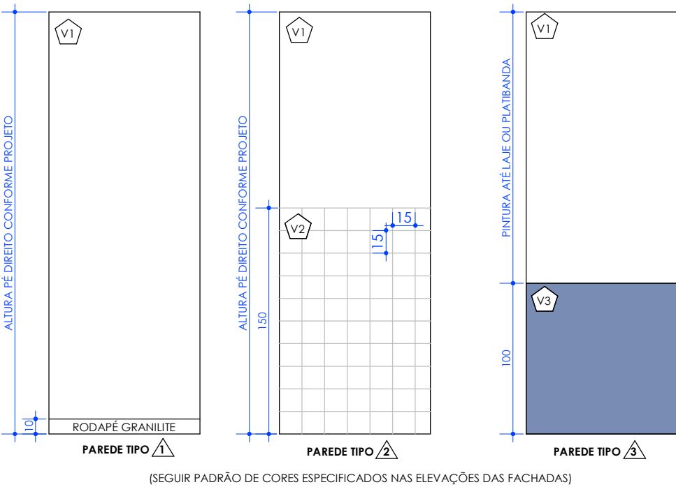
LEGENDA - ACABAMENTOS DE PAREDES (ARQ-QUADRO DE ACABAMENTOS)
