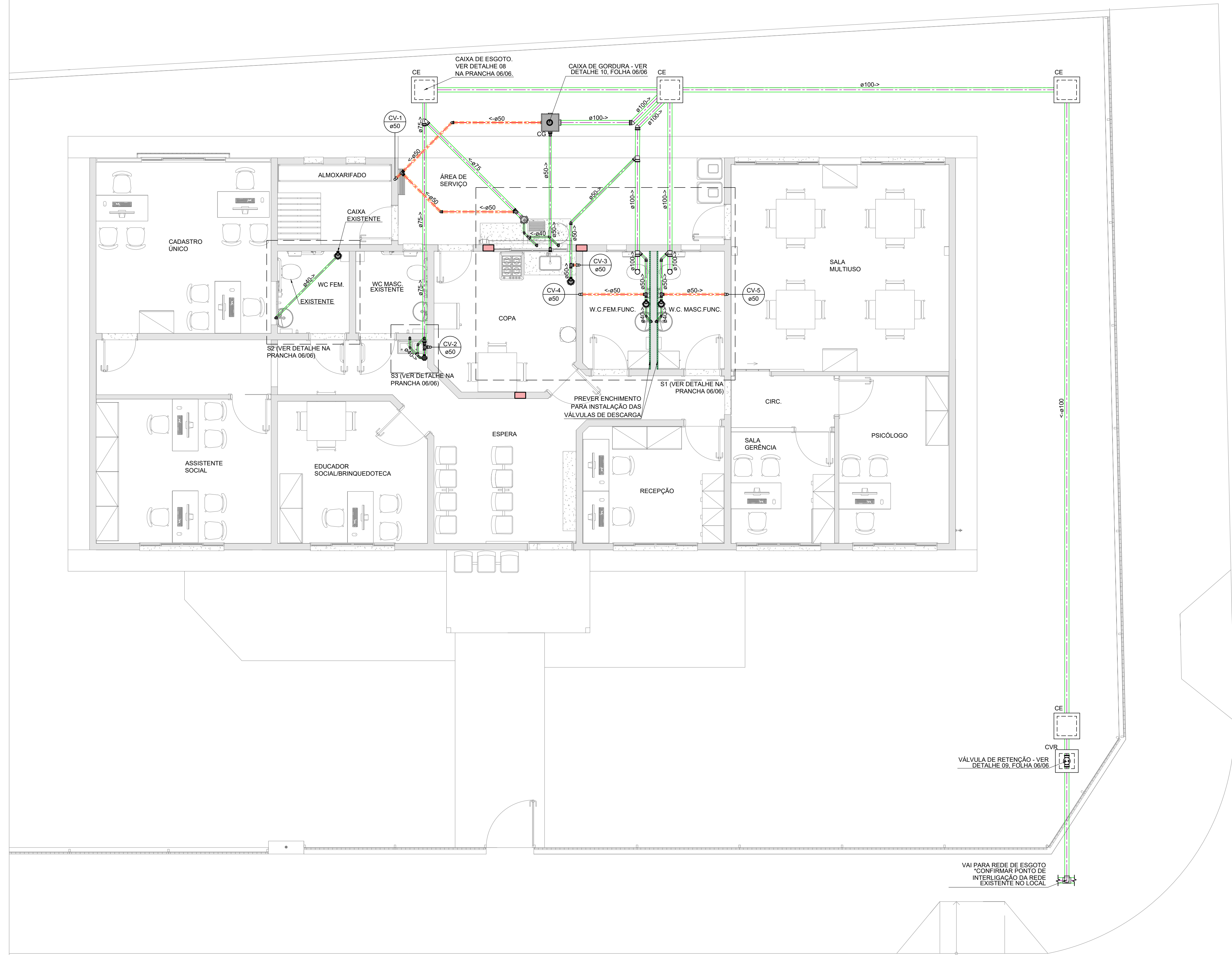
PLANTA BAIXA TÉRREO ESC.: 1/50
