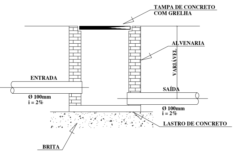
CORTE DA CAIXA DE INSPEÇÃO sem escala
