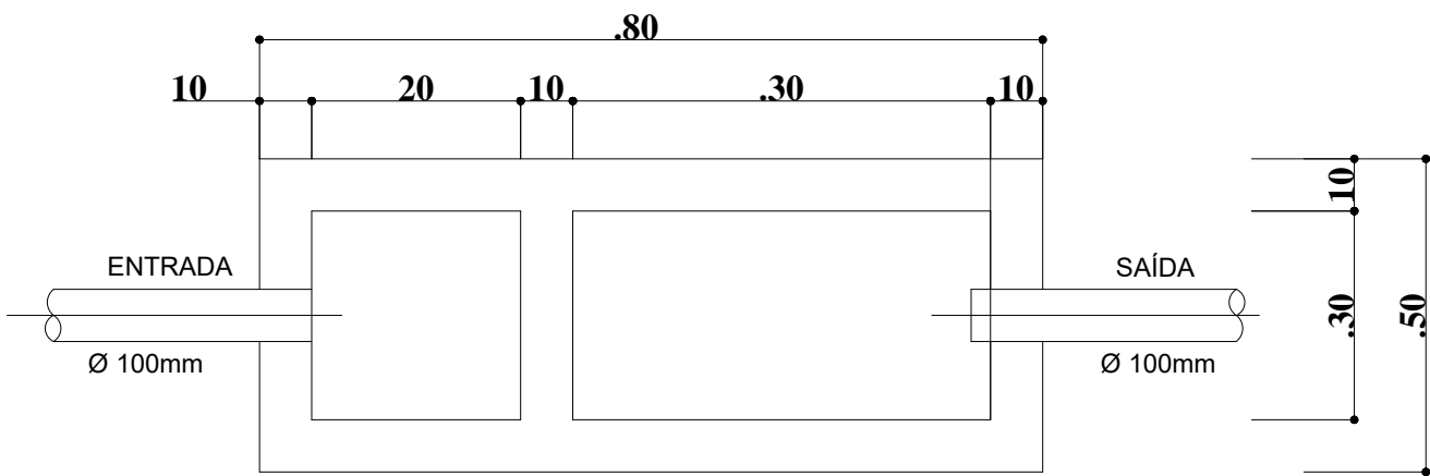
CAIXA DE GORDURA sem escala
