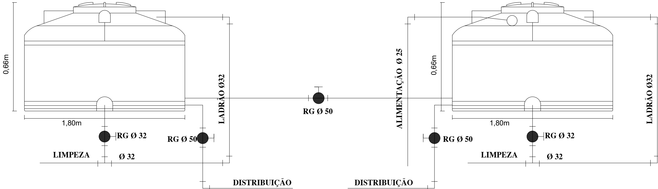
DETALHE CAIXA D'AGUA sem escala
