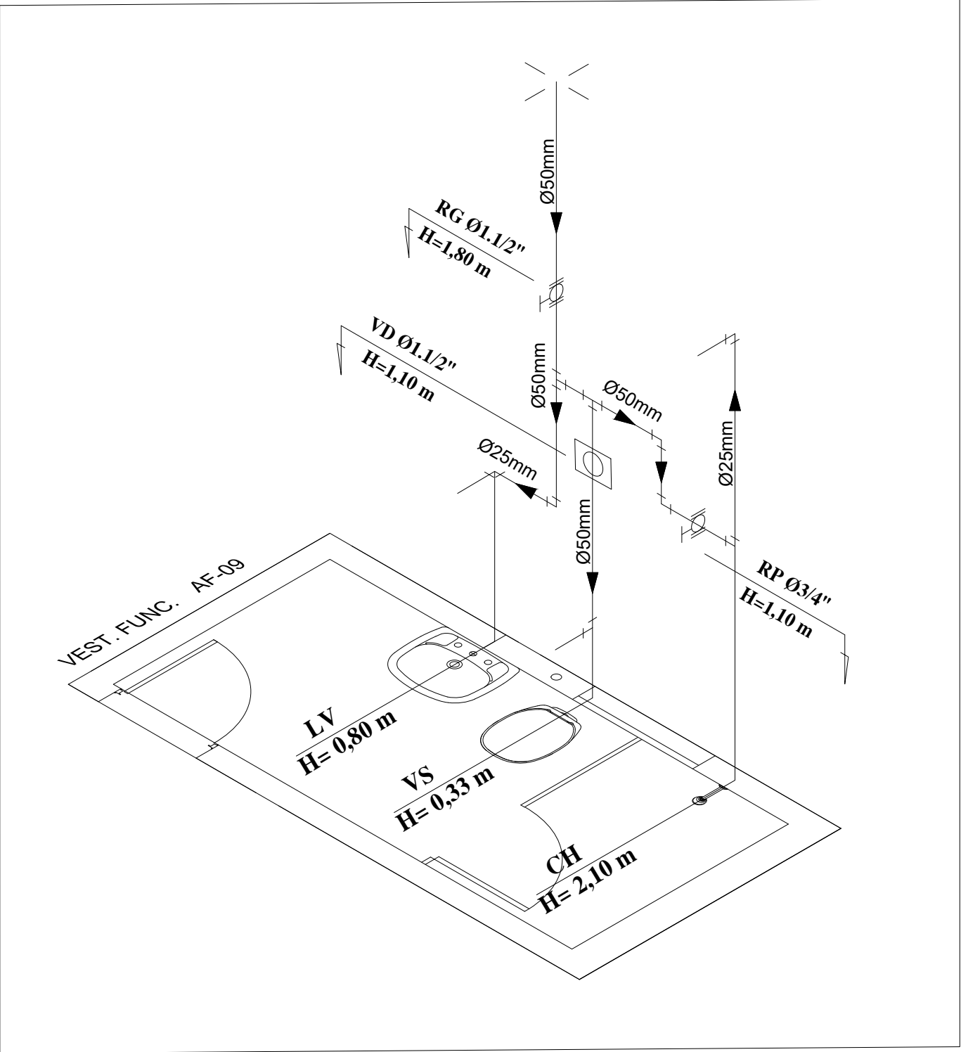
ISOMÉTRICO - VESTIÁRIO FUNCIONÁRIOS ESCALA _____ 1:25
