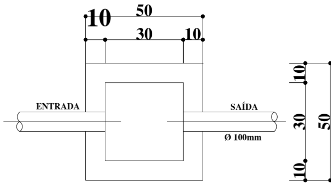
CAIXA DE INSPEÇÃO sem escala
