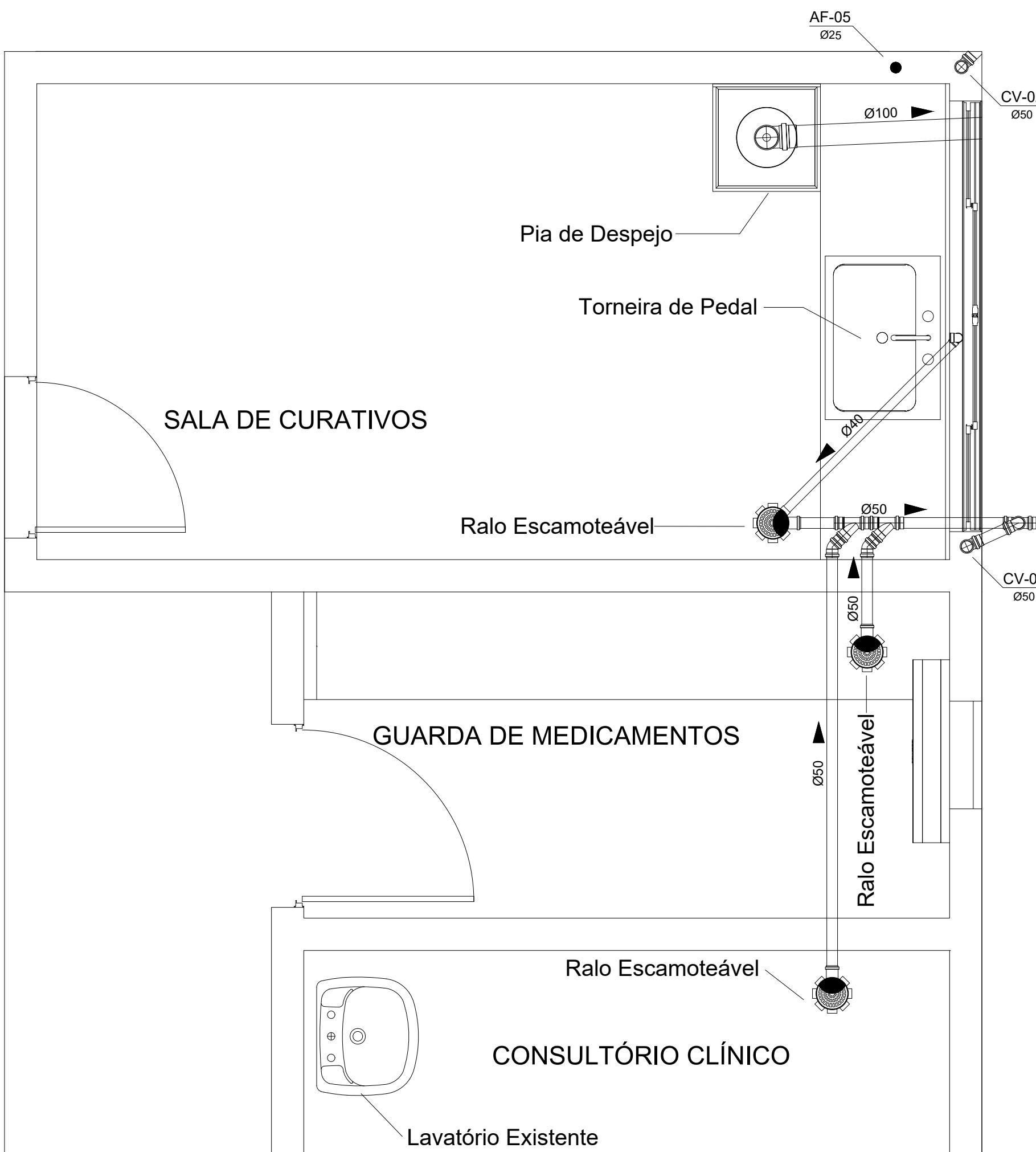
DETALHE - SALA DE CURATIVOS, GUARDA DE MEDICAMENTOS E CONSULTÓRIO CLÍNICO ESCALA 1:25
