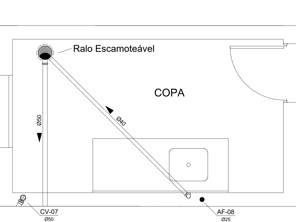
DETALHE - COPA ESCALA 1:25
