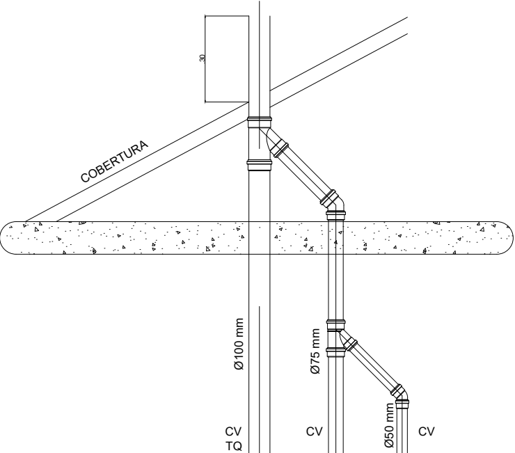
DET. COLUNA DE VENTILAÇÃO sem escala
