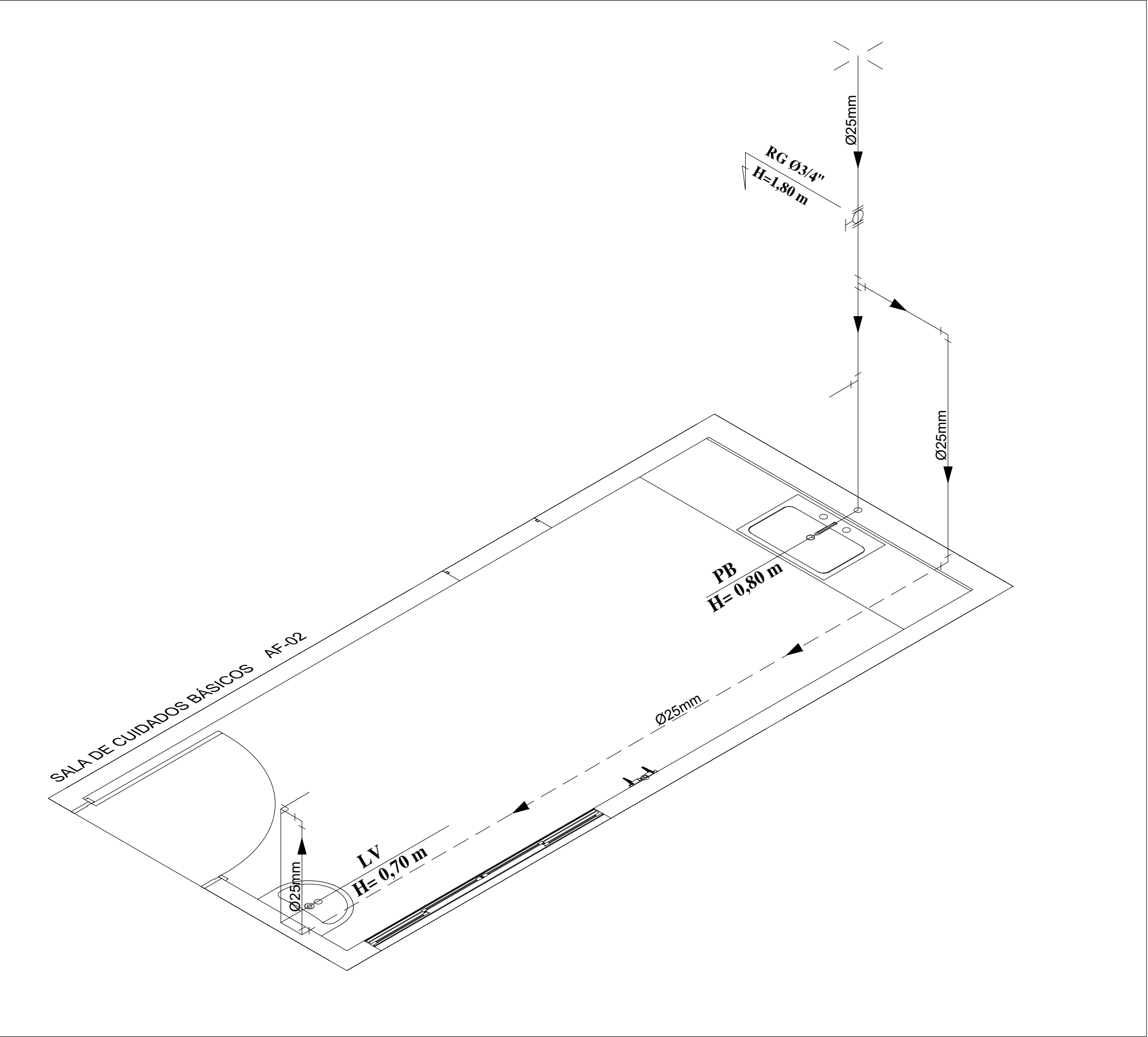
ISOMÉTRICO - SALA DE CUIDADOS BÁSICOS ESCALA 1:25
