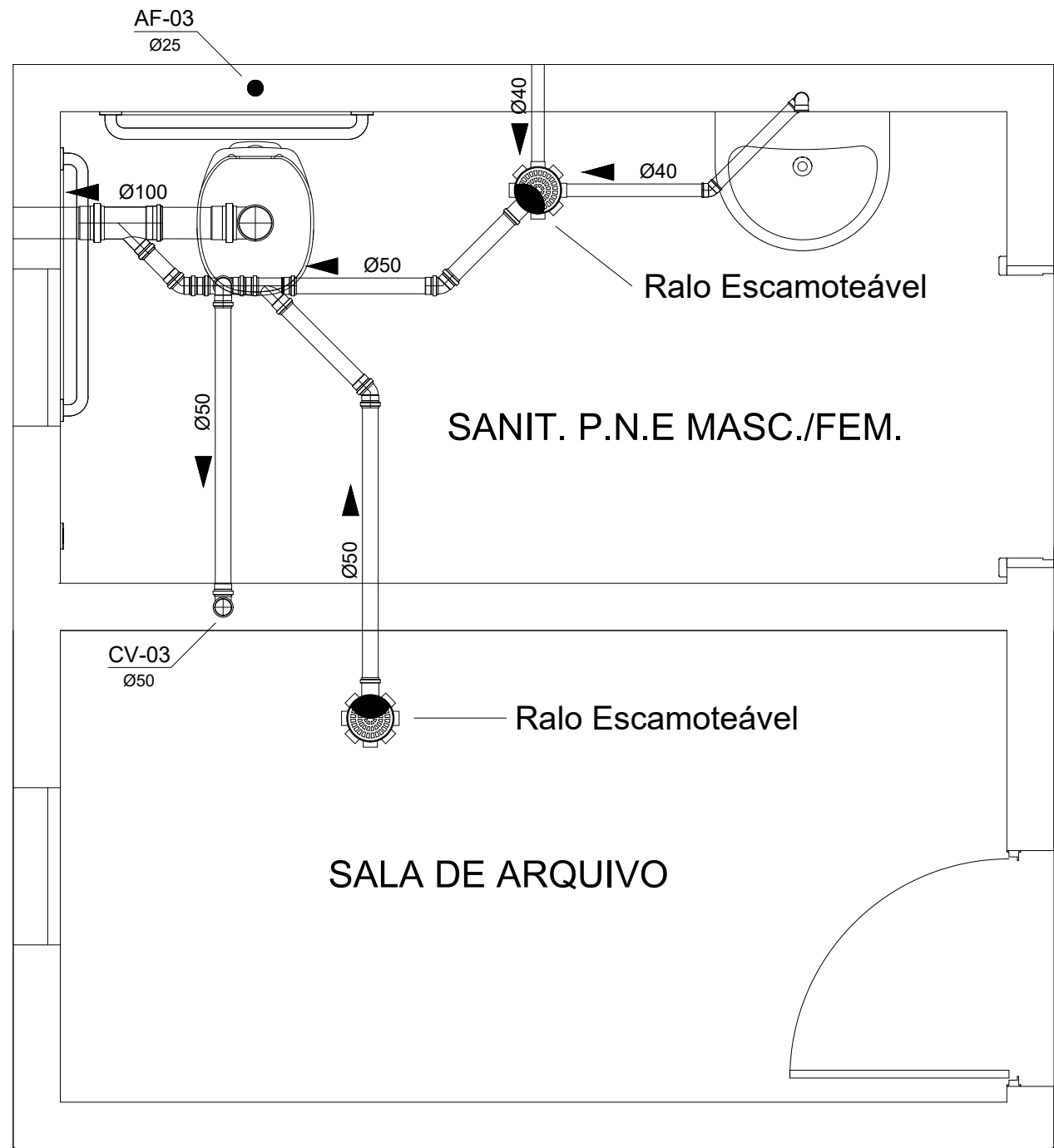
ISOMÉTRICO - SANIT. P.N.E. MAS./ FEM. E SALA DE ARQUIVO ESCALA 1:25
