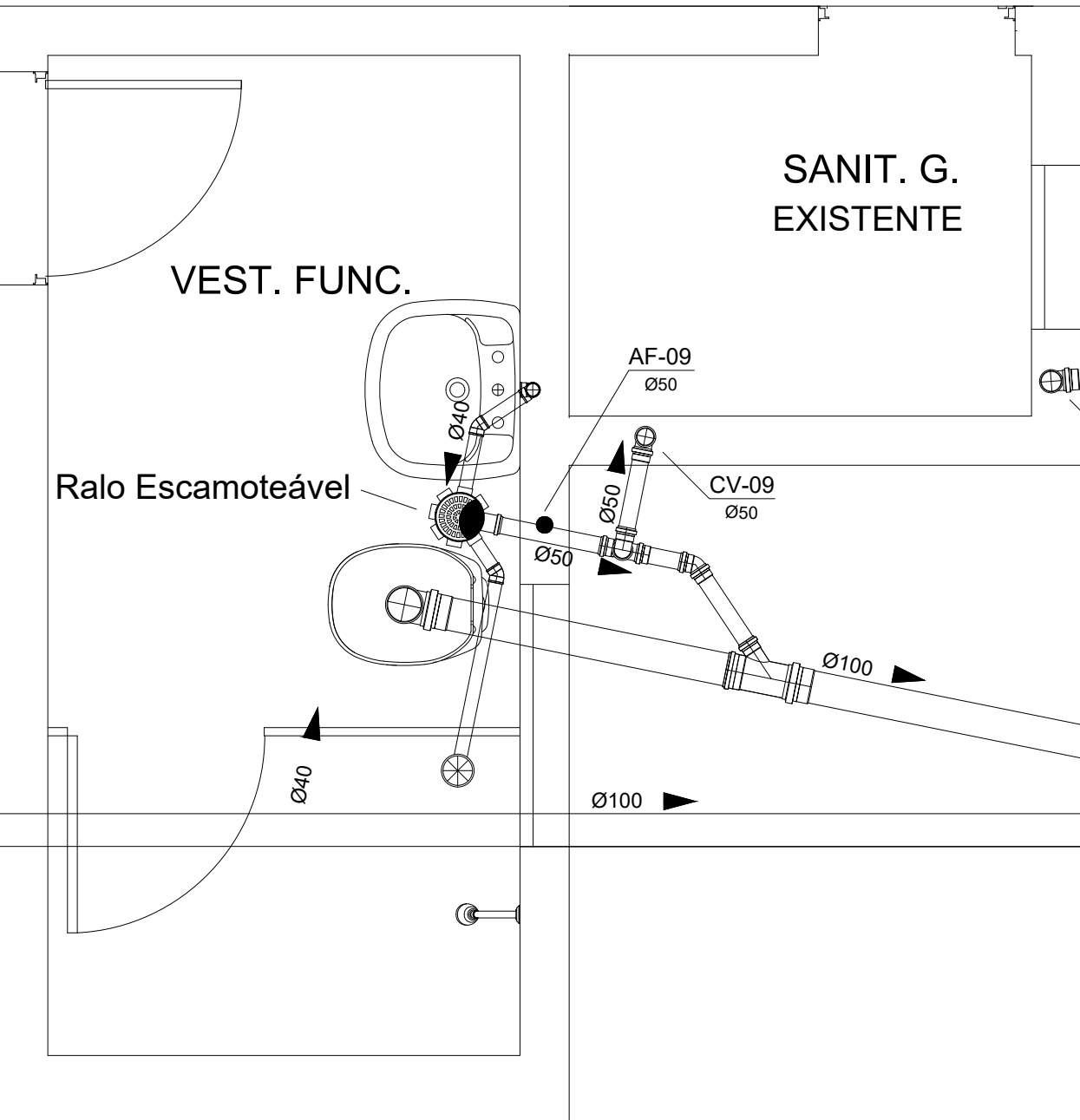
ISOMÉTRICO - VESTIÁRIO FUNCIONÁRIOS ESCALA 1:25
