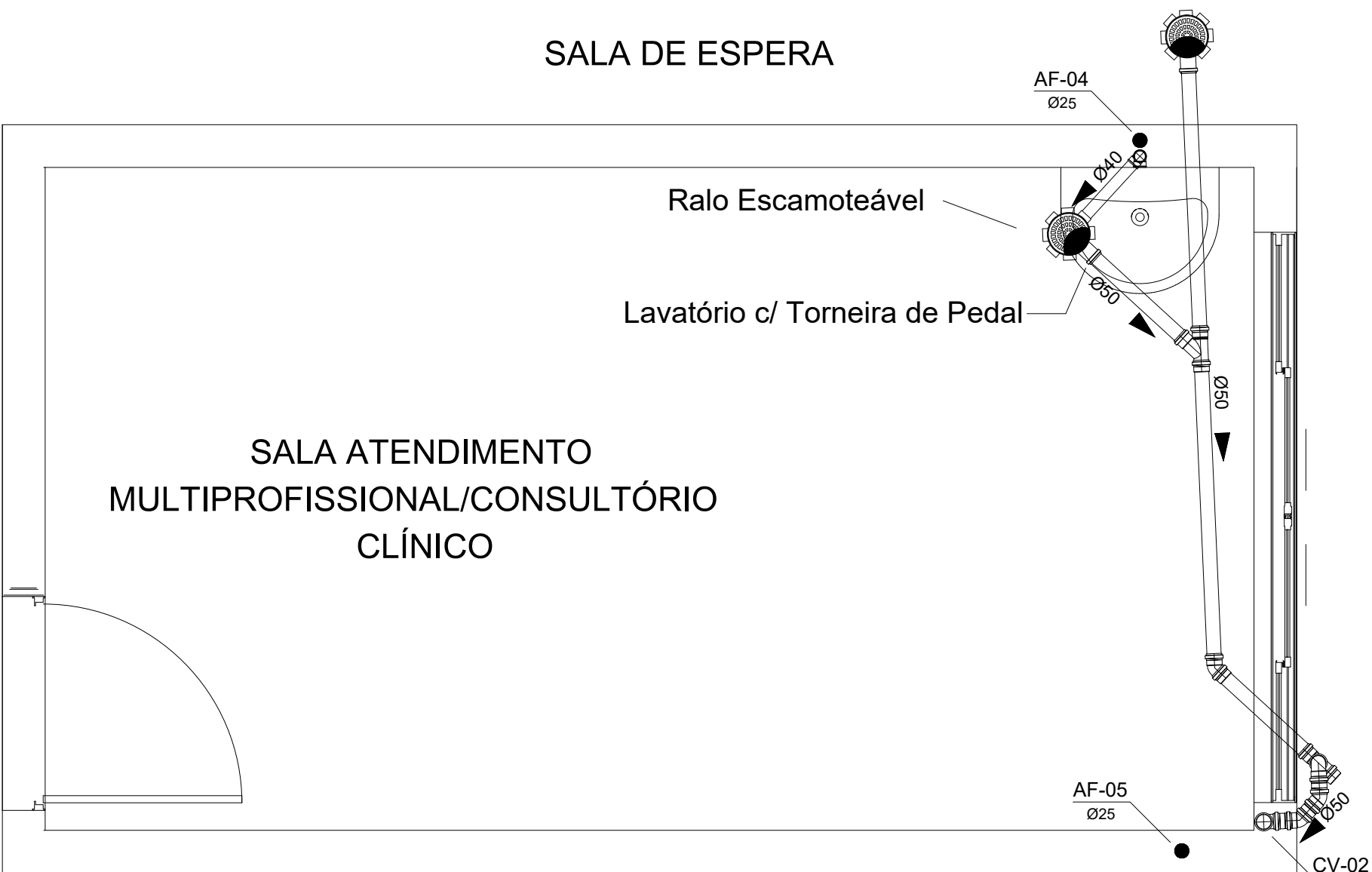
DETALHE - SALA ATENDIMENTO MULTIPROFISSIONAL/ CONSULTÓRIO CLÍNICO ESCALA 1:25
