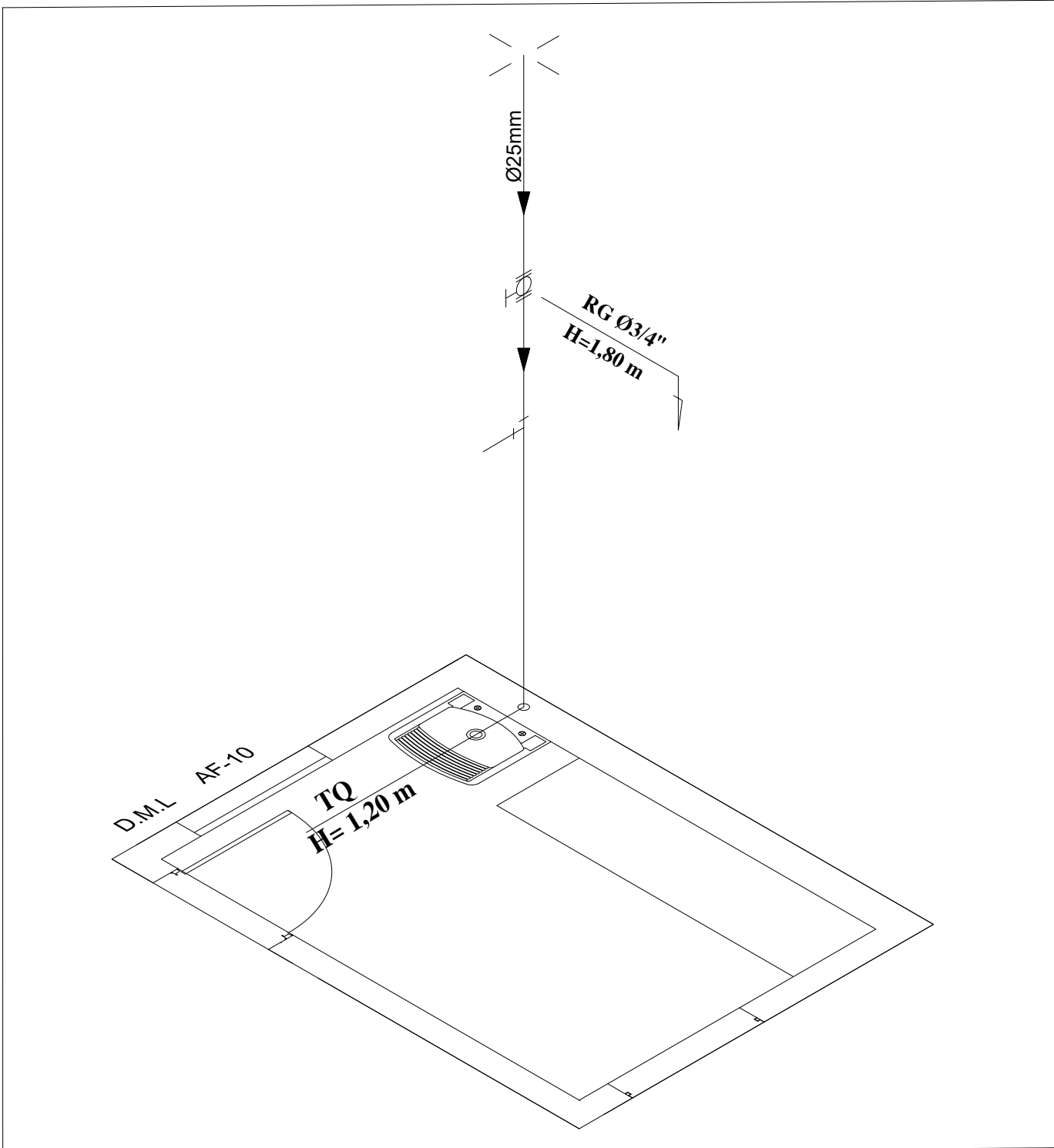
ISOMÉTRICO - D.M.L. ESCALA _____ 1:25
