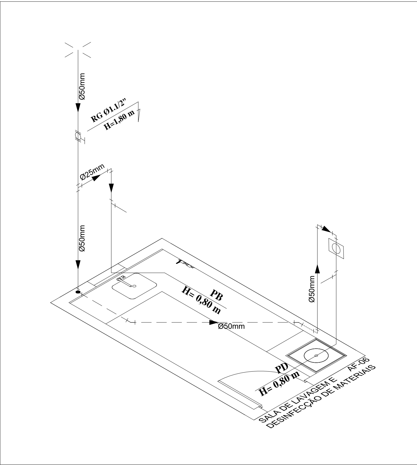
ISOMÉTRICO - SALA DE LAVAGEM E DESINFECÇÃO DE MATERIAIS ESCALA _____ 1:25
