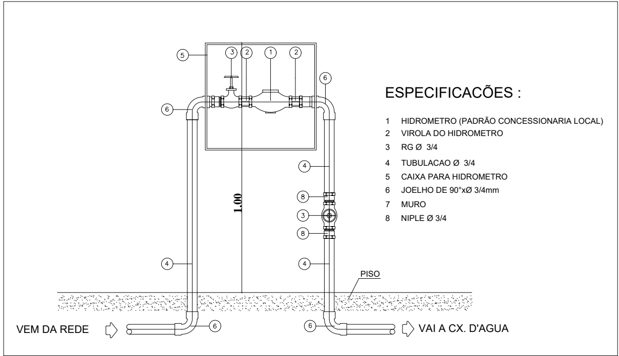
DET. INSTALAÇÃO DO HIDROMETRO sem escala
