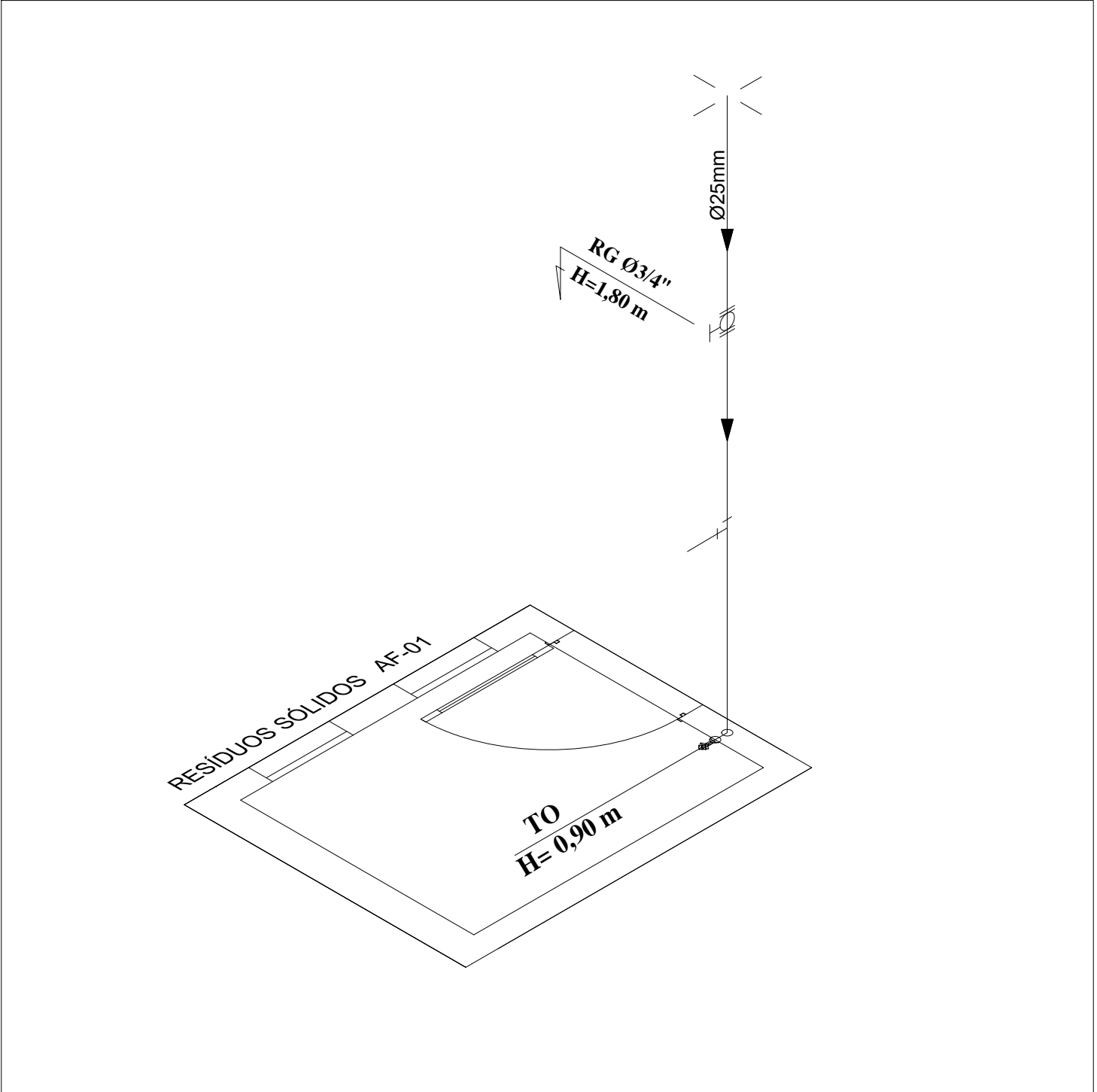
ISOMÉTRICO - RESÍDUOS SÓLIDOS ESCALA 1:25
