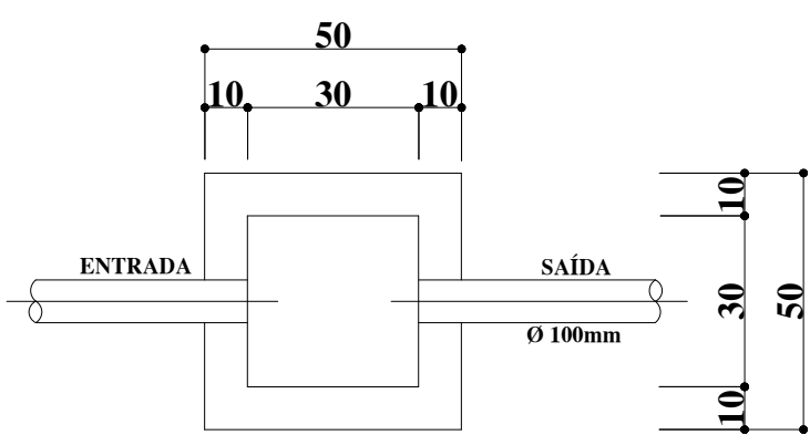
CAIXA DE AREIA sem escala
