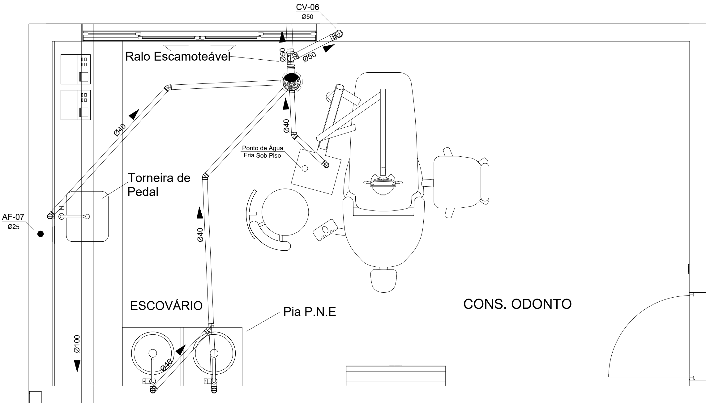
DETALHE - CONSULTÓRIO ODONTO/ESCOVÁRIO ESCALA 1:25
