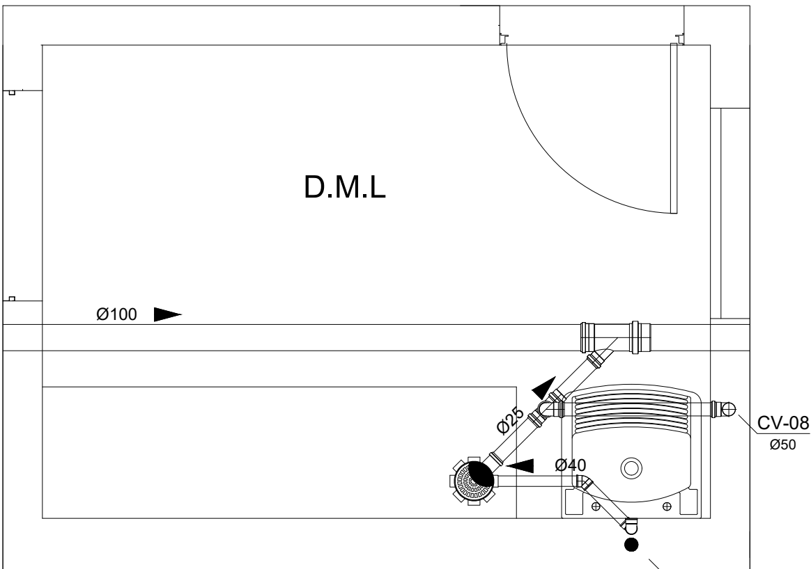
DETALHE - D.M.L. ESCALA 1:50
