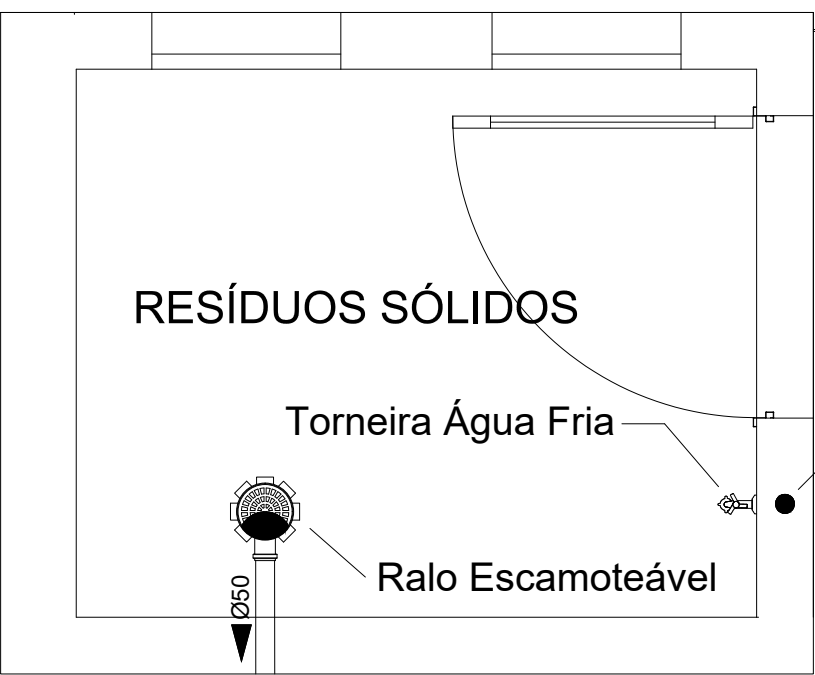
DETALHE - RESÍDUOS SÓLIDOS ESCALA 1:25
