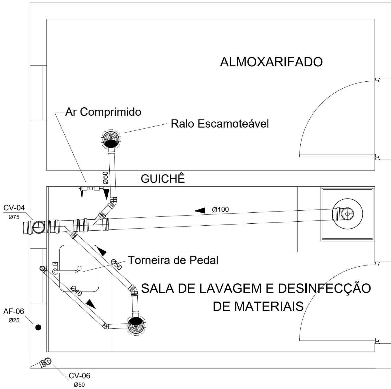
DETALHE - SALA DE LAVAGEM E DESINFECÇÃO DE MATERIAIS ESCALA 1:25
