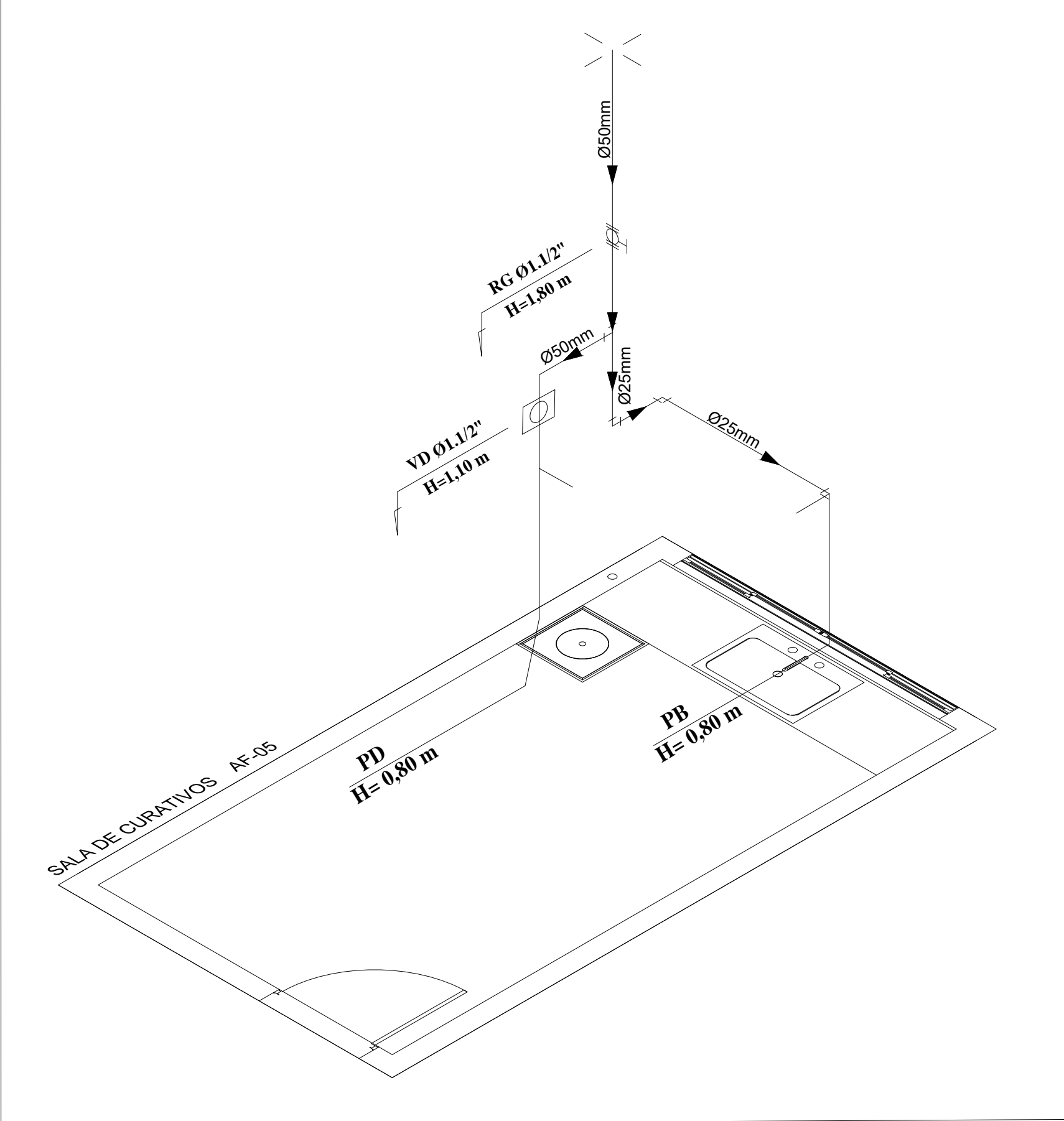
ISOMÉTRICO - SALA DE CURATIVOS ESCALA 1:25
