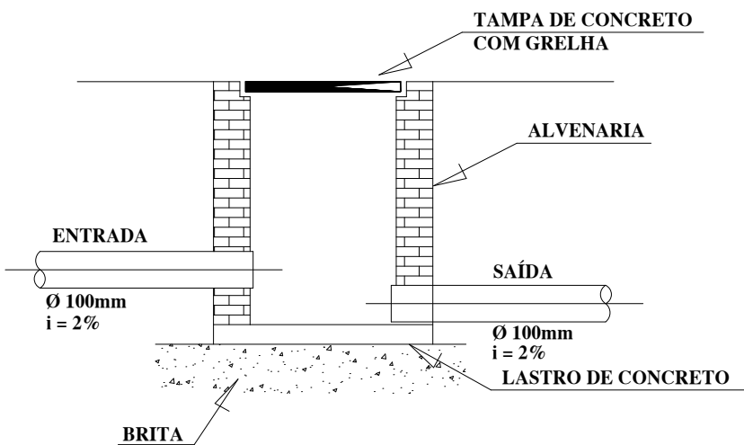
CORTE DA CAIXA DE AREIA sem escala
