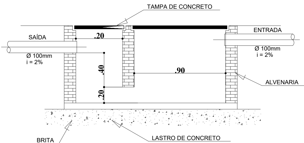
CORTE CAIXA DE GORDURA sem escala
