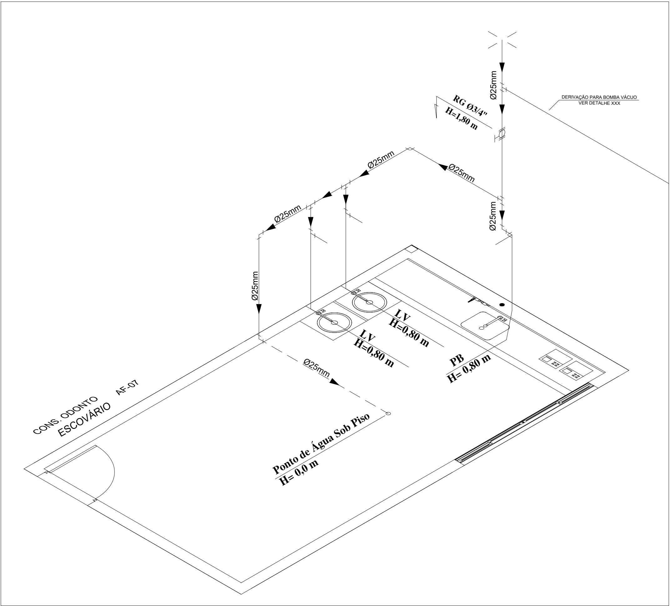
ISOMÉTRICO - CONSULTÓRIO ODONTO/ESCOVÁRIO ESCALA _____ 1:25
