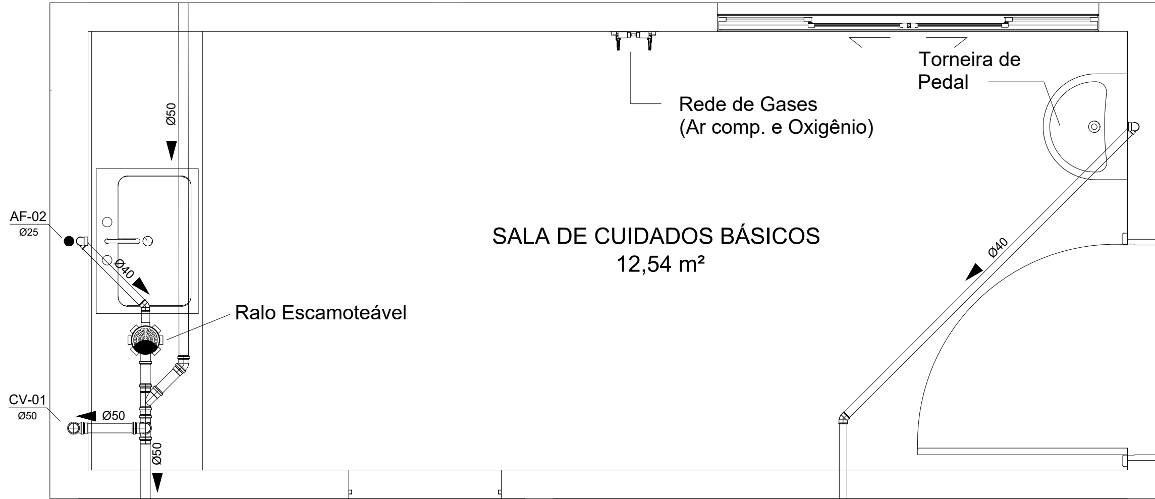
DETALHE - SALA DE CUIDADOS BÁSICOS ESCALA 1:25
