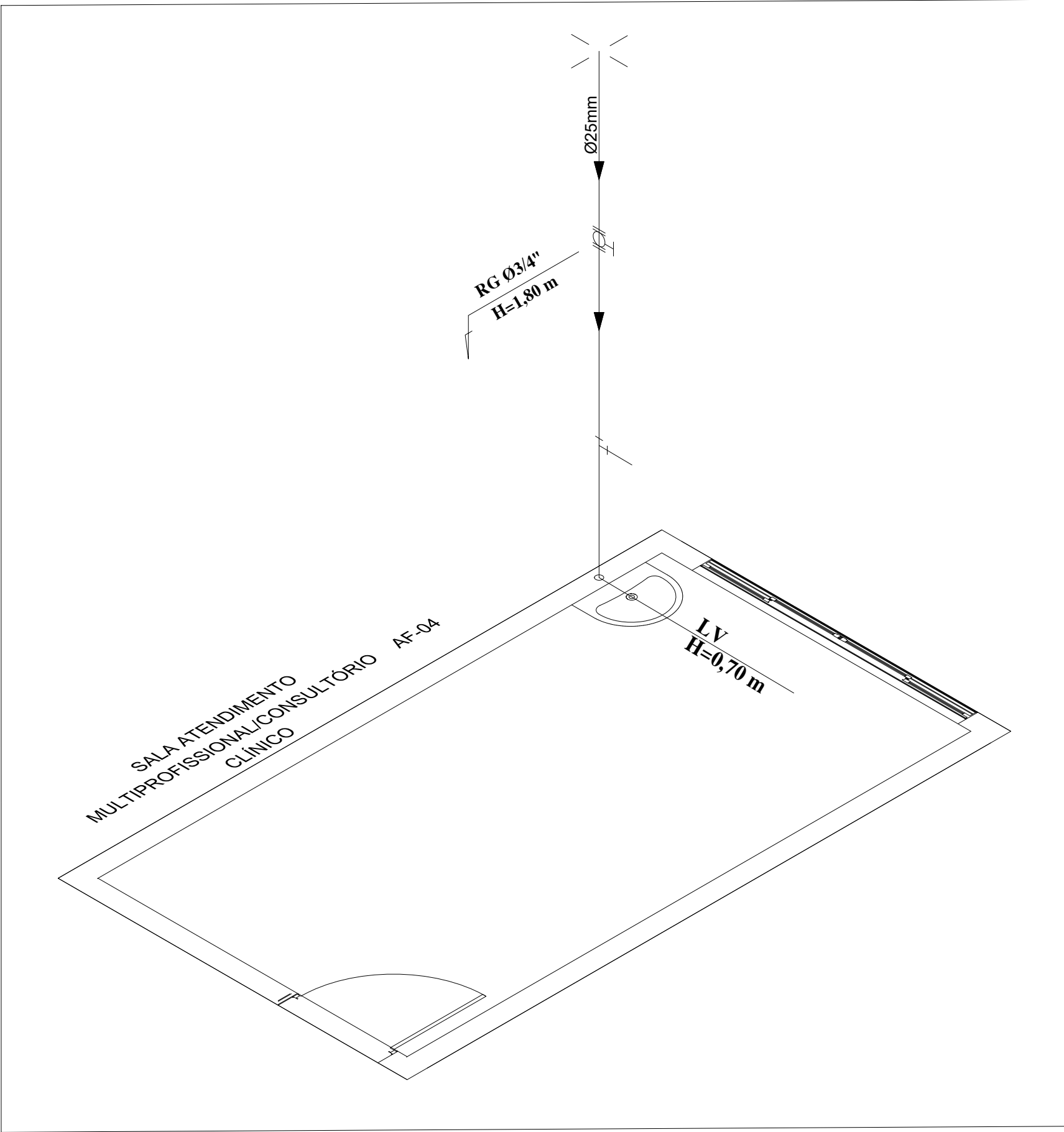
ISOMÉTRICO - SALA ATENDIMENTO MULTIPROFISSIONAL/ CONSULTÓRIO CLÍNICO ESCALA 1:25
