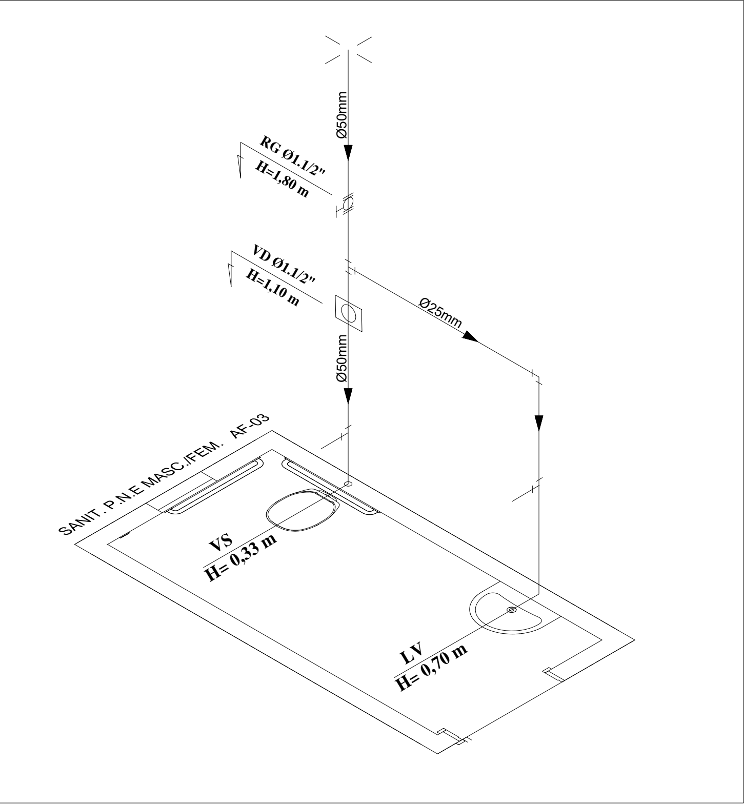
ISOMÉTRICO - SANIT. P.N.E. MAS./ FEM. ESCALA 1:25
