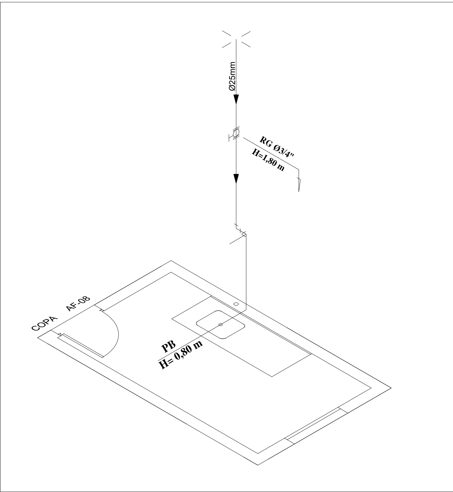
ISOMÉTRICO - COPA ESCALA _____ 1:25
