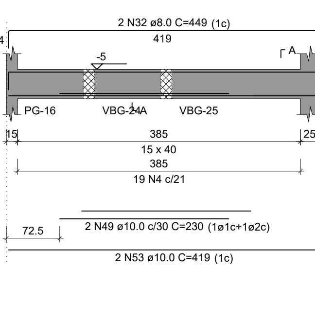
VBG-12 ESC 1:50
