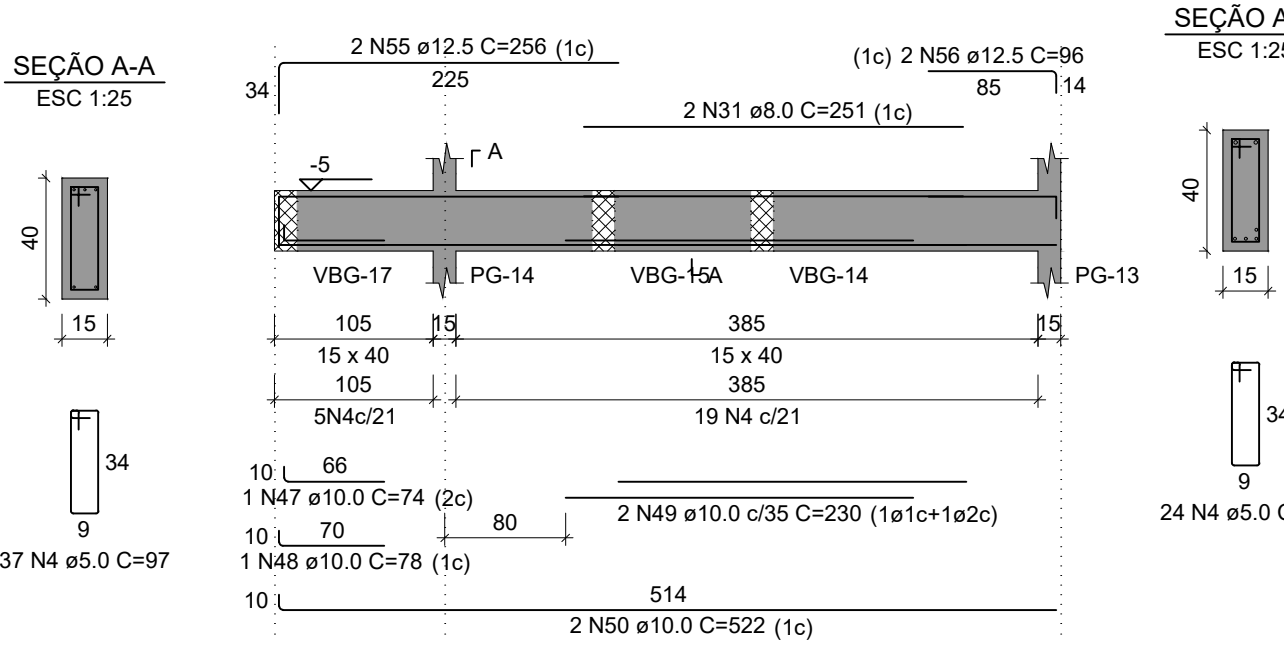
VBG-14 ESC 1:50
