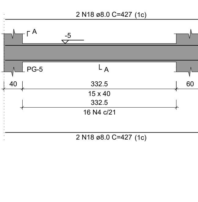
VBG-4 ESC 1:50
