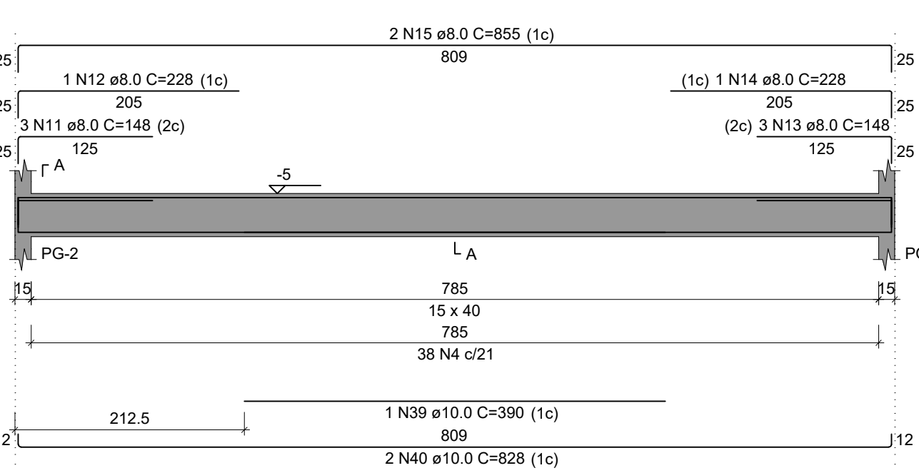
VBG-6 ESC 1:50
