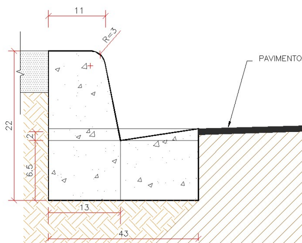
Figura 2 – Meio fio com sarjeta.
