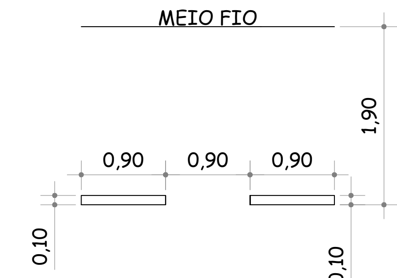
DETALHE FAIXA TRACEJADA BRANCA
