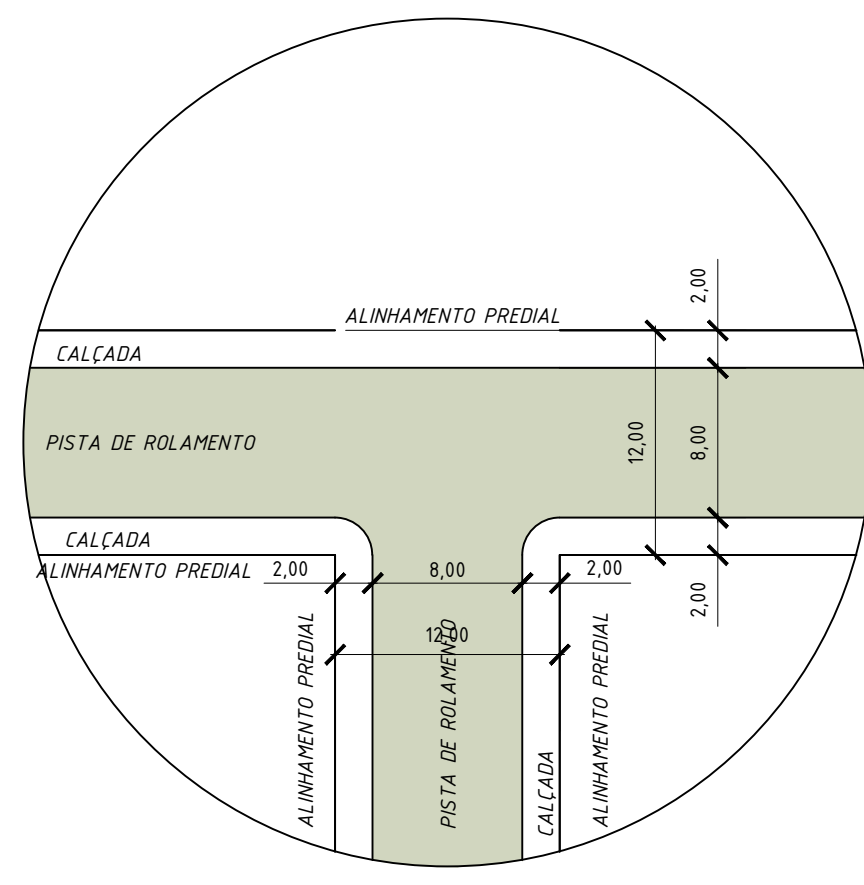
DET. TÍPICO DOS CRUZAMENTOS ESCALA 1 / 500
