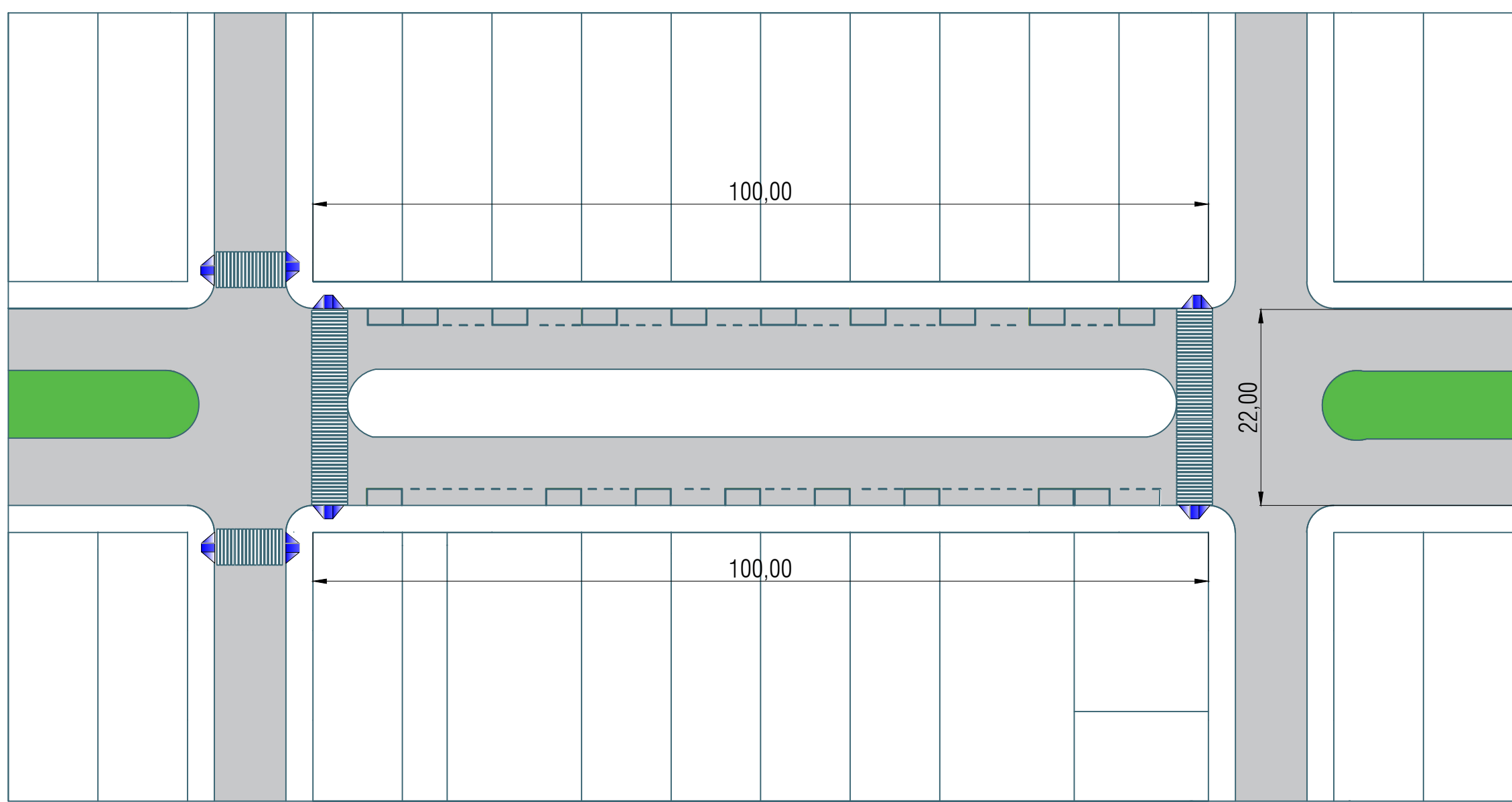
TRECHO TIPO 02 ESC. 1/1000
