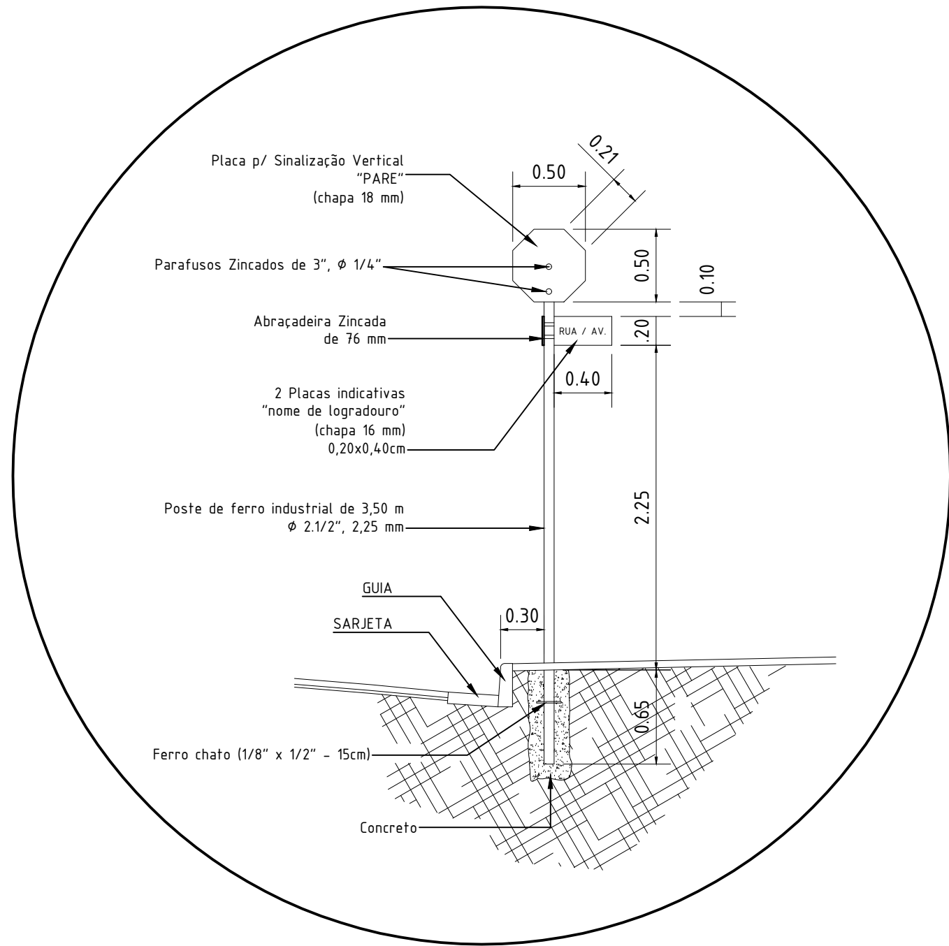
DET. TÍPICO DOS CRUZAMENTOS ESCALA 1 / 500
