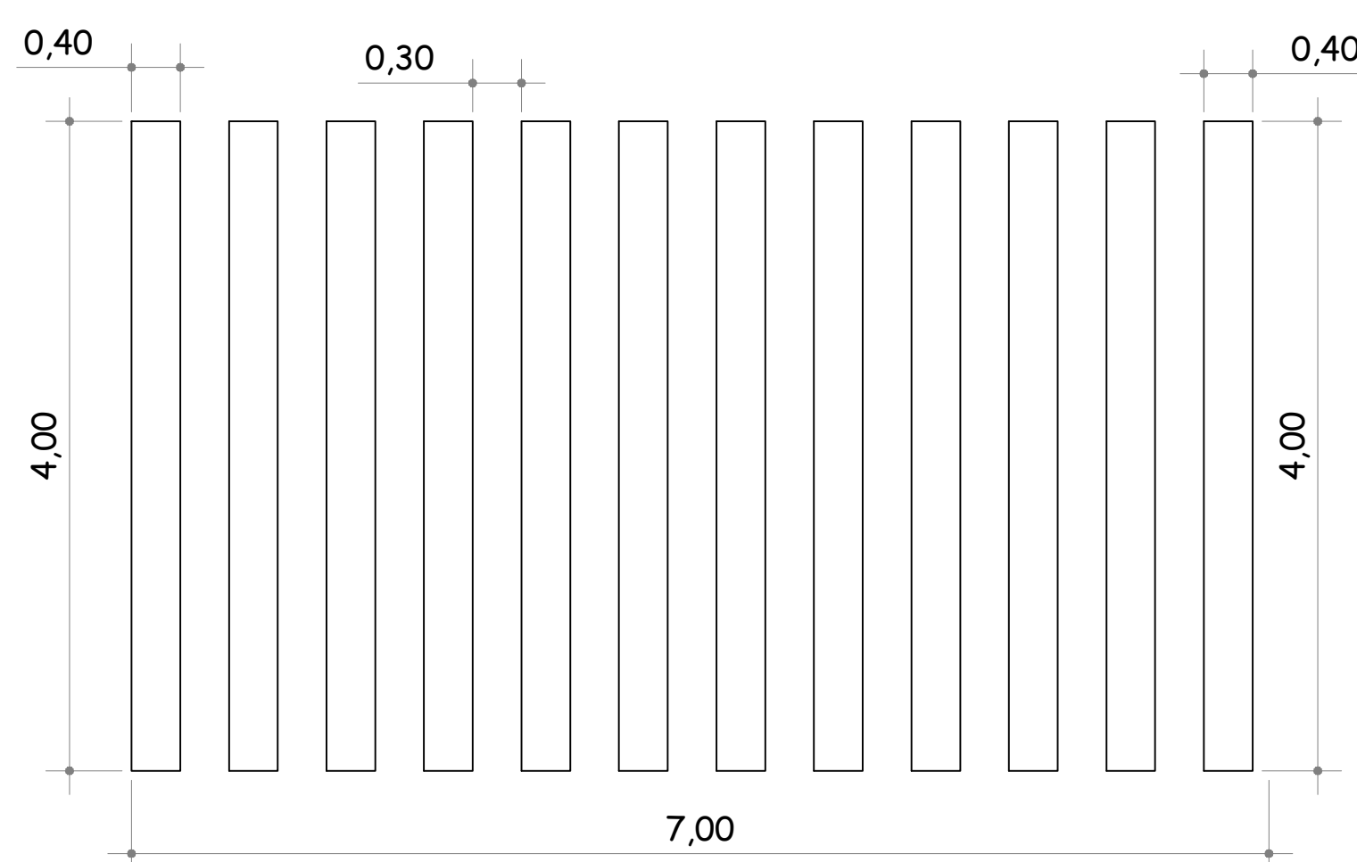
DETALHE FAIXA PEDESTRE BRANCA 3,00
