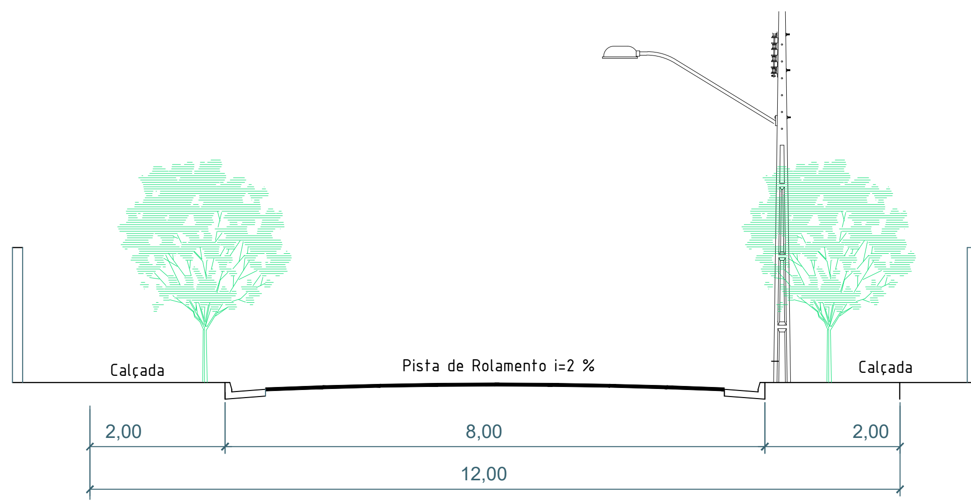
DETALHE DA AVENIDAS/RUAS DE 12,00 - METROS ESCALA 1 / 100
