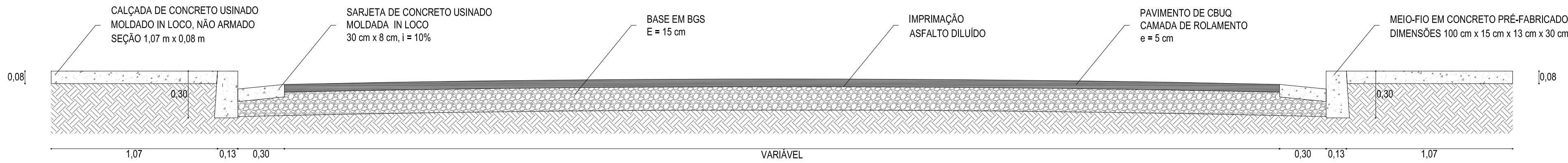
SEÇÃO TRANSVERSAL DA VIA NO TRECHO 4 1:20
