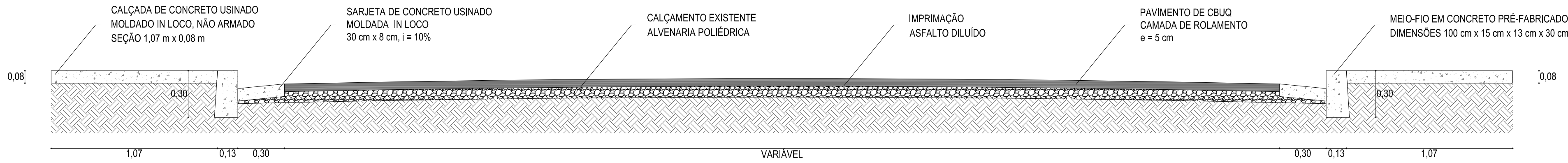
SEÇÃO TRANSVERSAL DA VIA NOS TRECHOS 1, 2 E 3 1:20
