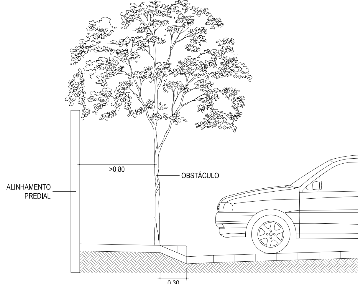
DETALHE DA CALÇADA 1:25
