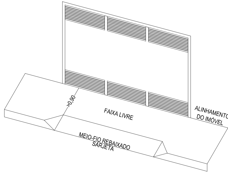
DETALHE DO ACESSO ÀS GARAGENS SEM ESCALA
