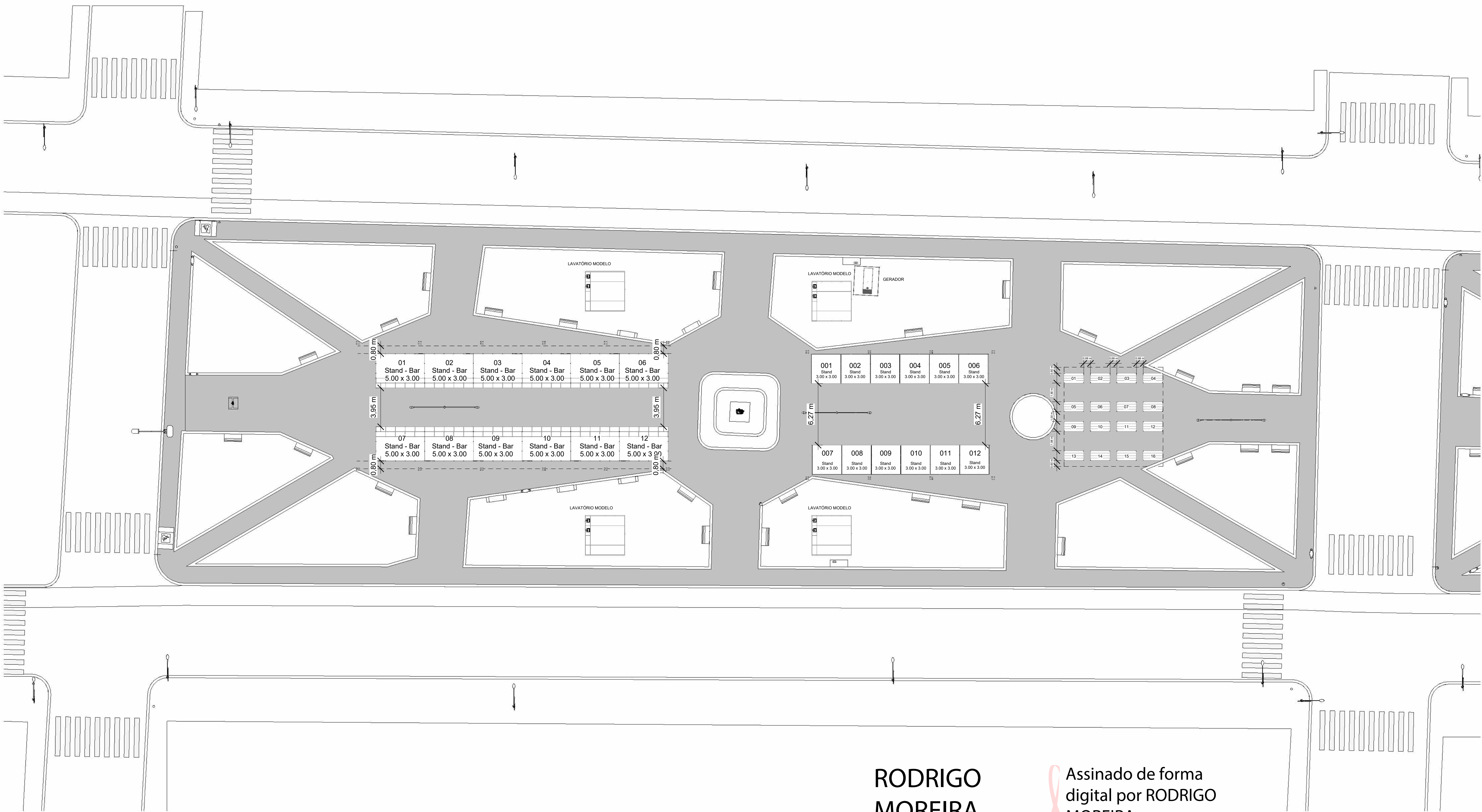
1 Panta Baixa 1 : 200
