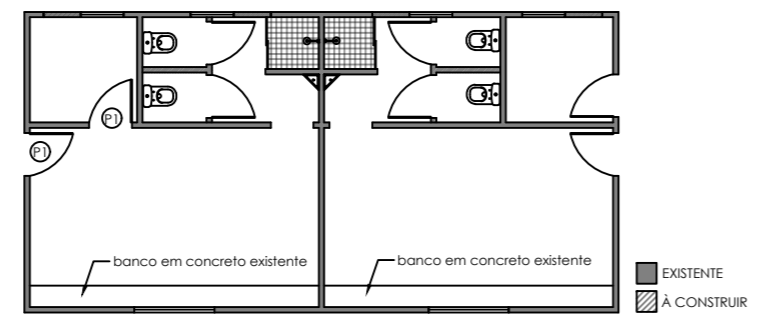
PLANTA LAYOUT esc 1:100
