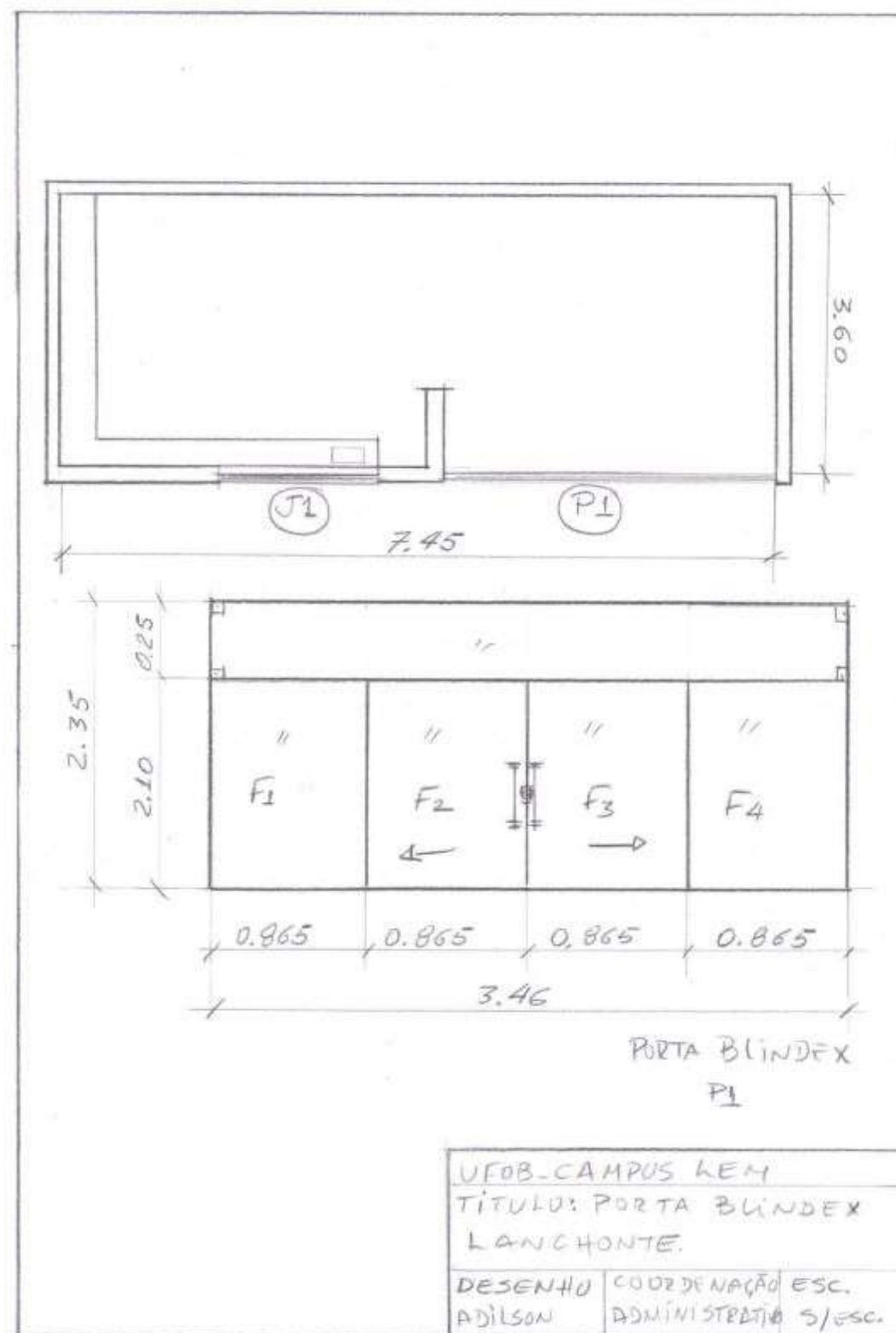
IMAGEM 03 - CROQUI - PORTA VIDRO BLINDEX
