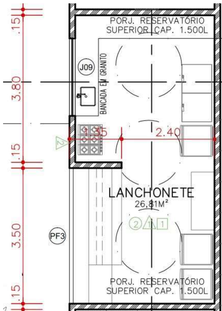
IMAGEM 02 - PLANTA BAIXA - IMAGEM AMPLIADA - LANCHONETE
