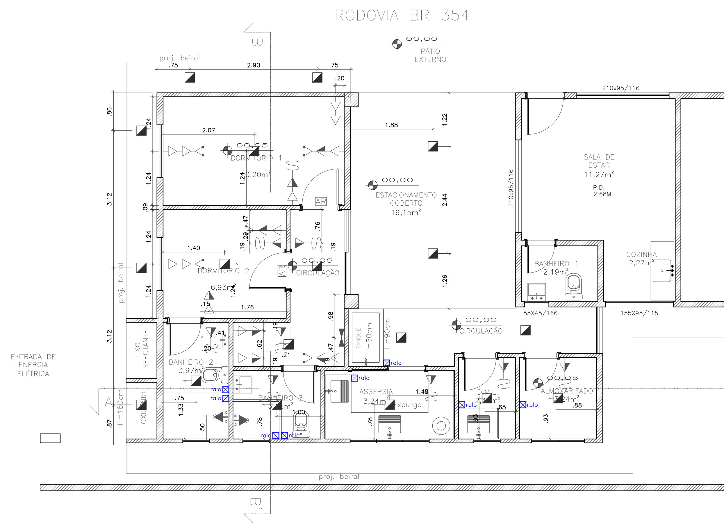
LUMINOTÉCNICO ESCALA: 1/50
