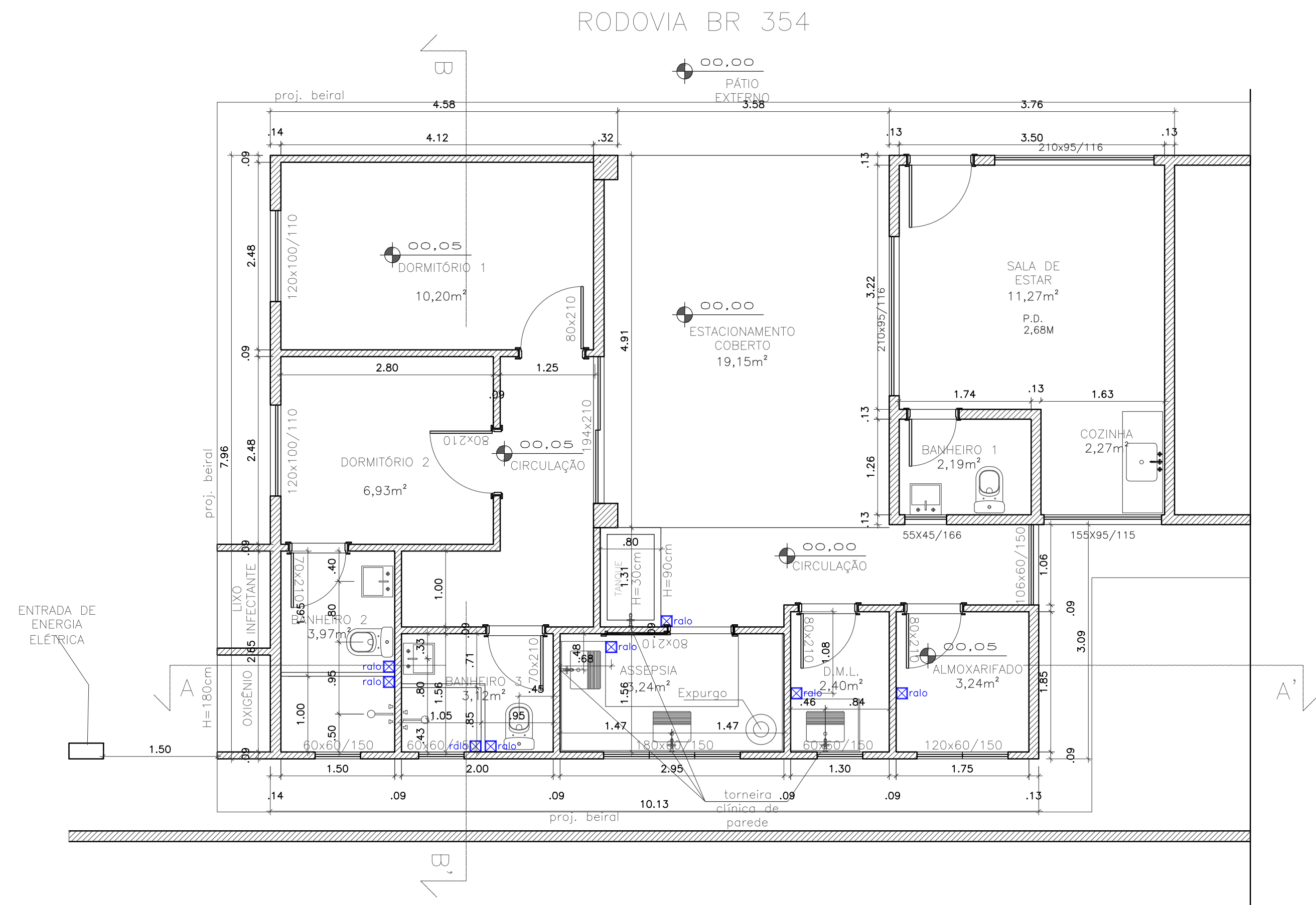
PLANTA BAIXA R01 ESCALA: 1/50
