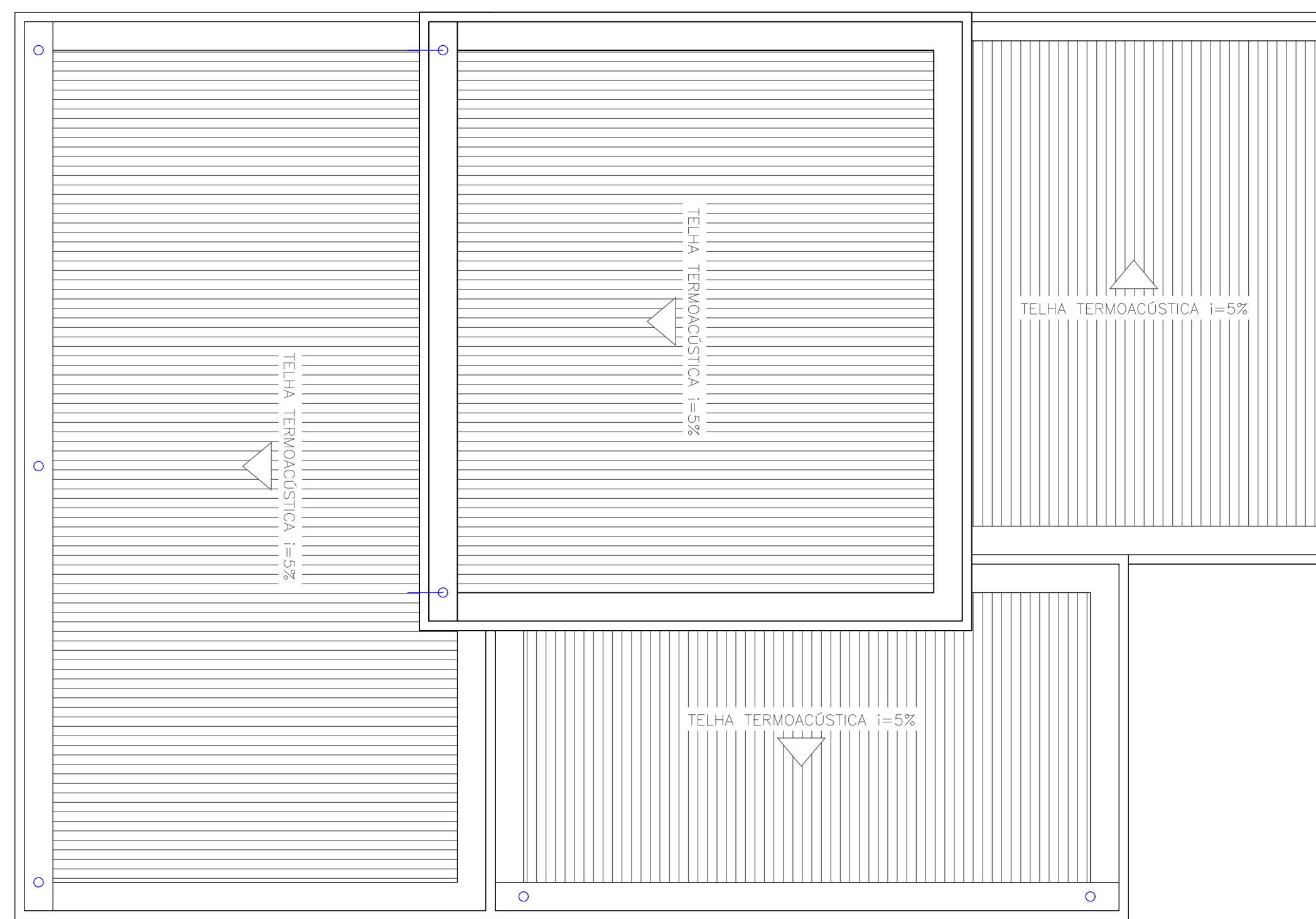
PLANTA DE COBERTA ESCALA: 1/100
