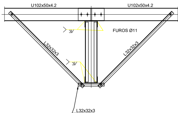
DETALHE DA MÃO FRANCESA
