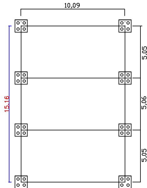
PLANTA DE Fôrma FUNDAÇÃO esc: 1/100
