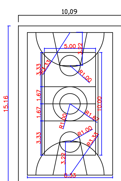
PLANTA BAIXA esc: 1/100
